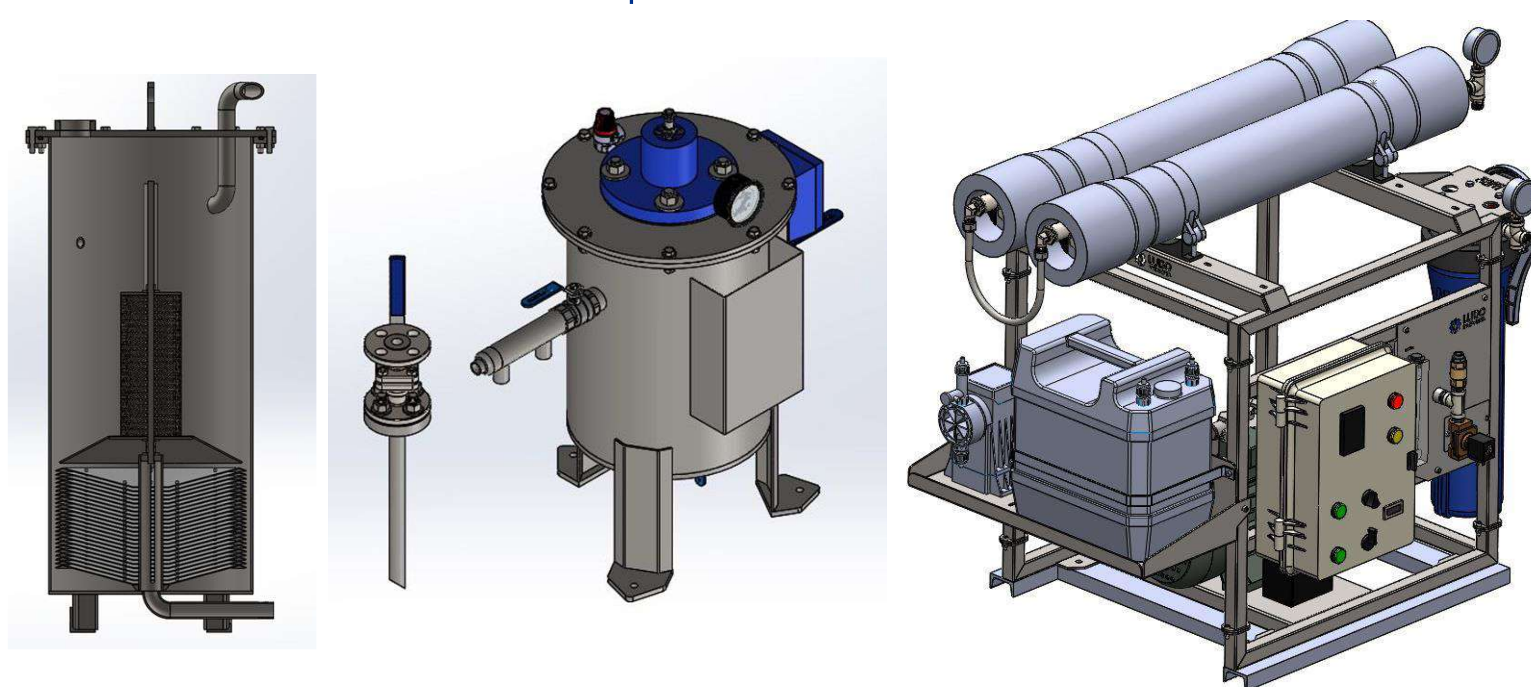
Diferentes vistas de algunos de los componentes y equipos diseñados
