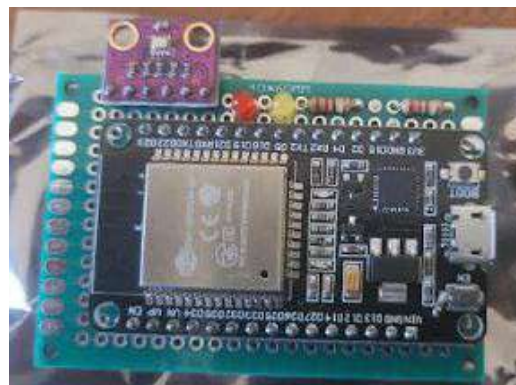
Kit didáctico IoT.
