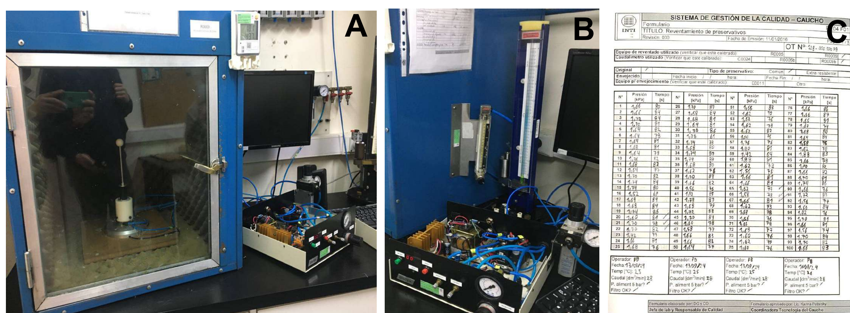
Figura 1: A) Cámara de reventado de preservativos. B) Controlador de equipo de reventado. C) Planilla de registro de datos primarios manual del ensayo de reventado de preservativos.
