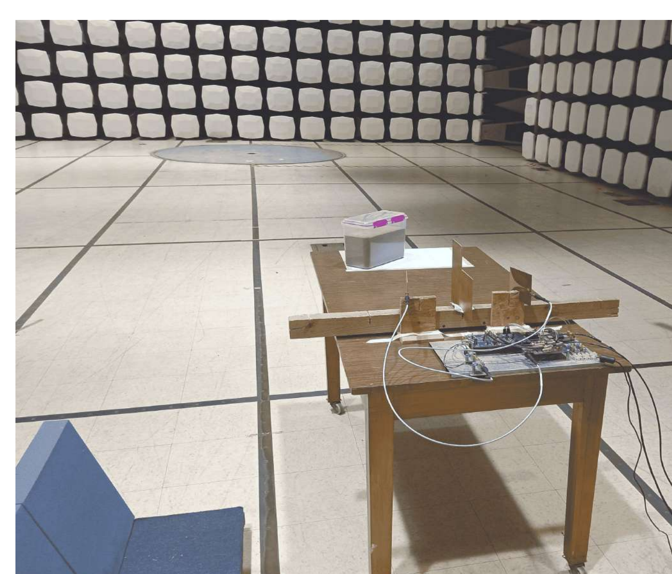
Setup de medición: Cámara semi-anechoica (izquierda), Clasificación (derecha).
