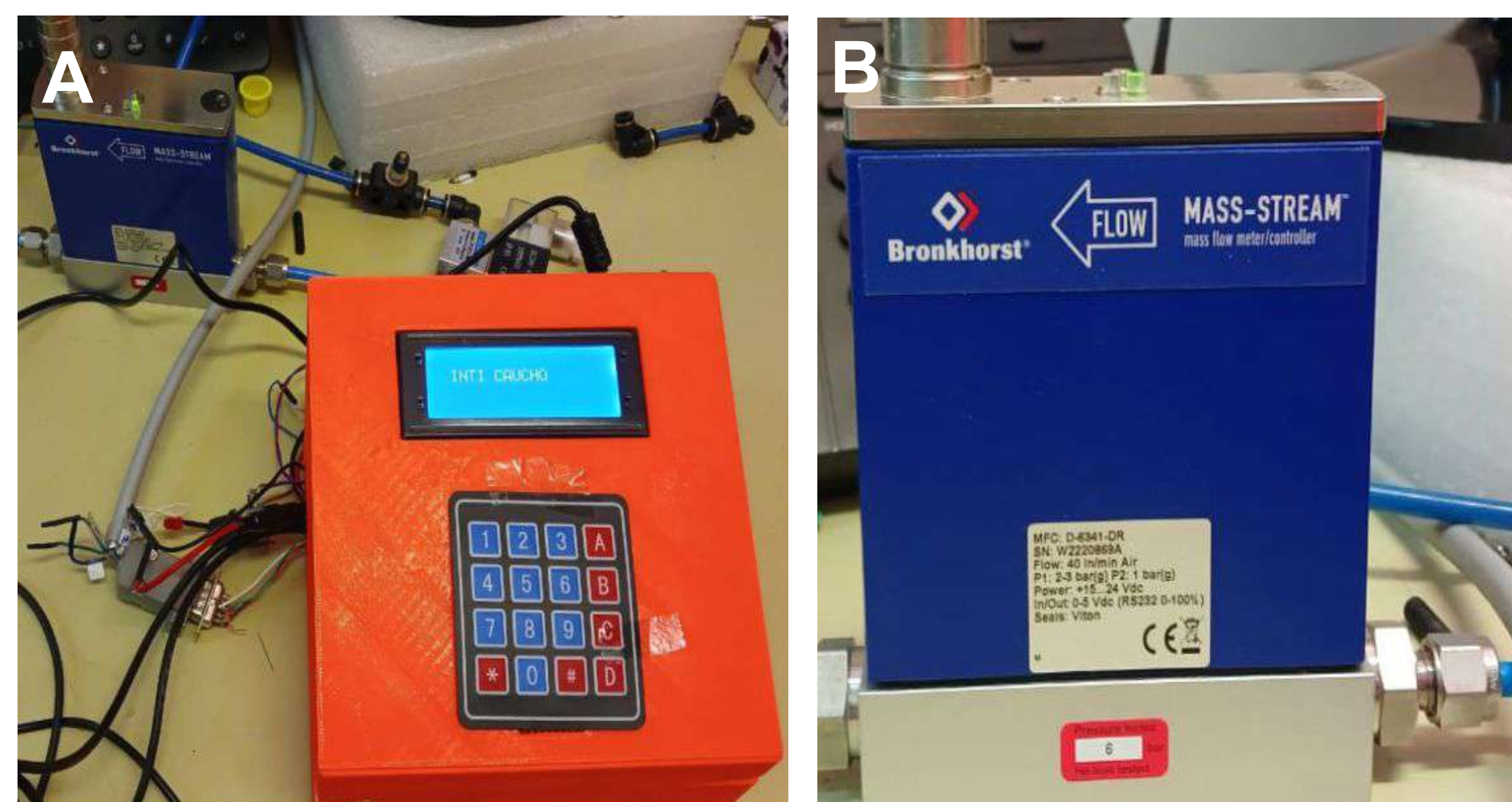
Figura 2: A) Display y controlador de ensayo. B) Caudalímetro másico digital.
