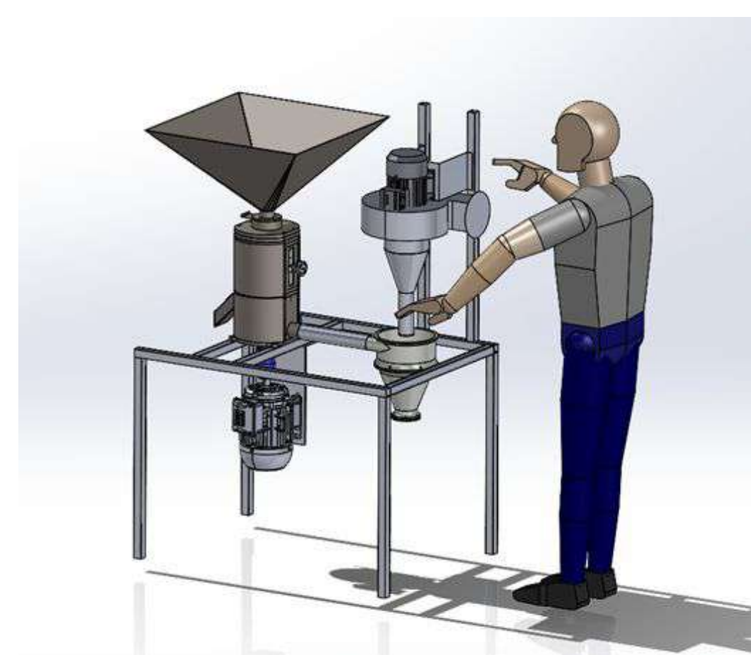
Diseño 3D del equipo a fabricar.
