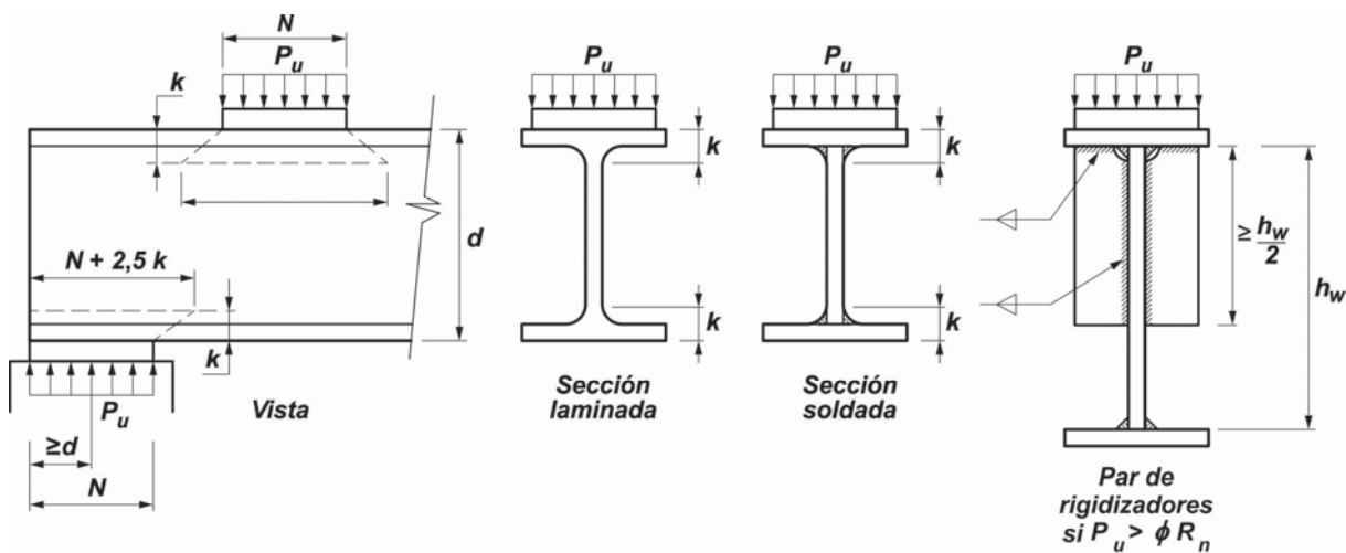
Figura J.10.2. Fluencia local del alma.
