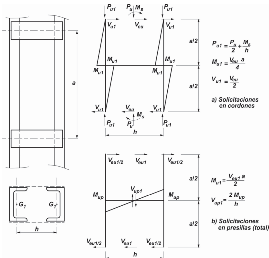
Figura E.6.8. Solicitaciones en cordones y presillas.
