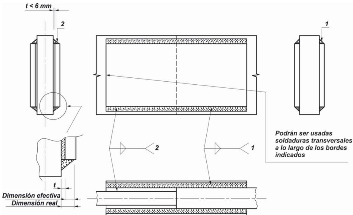
Figura J.5.1. Chapa de relleno con espesor menor que 6 mm.
