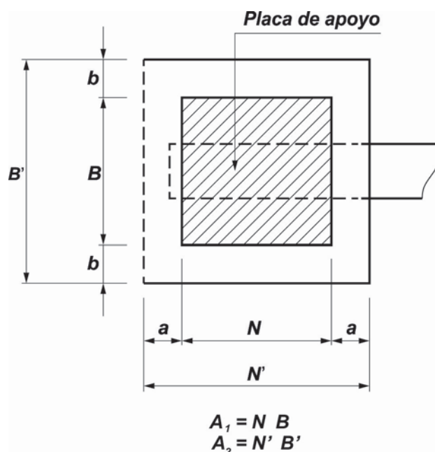
Figura J.9.1. Áreas de apoyo.
