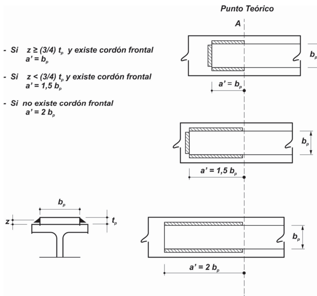
Figura F.13.1. Determinación de a' .
