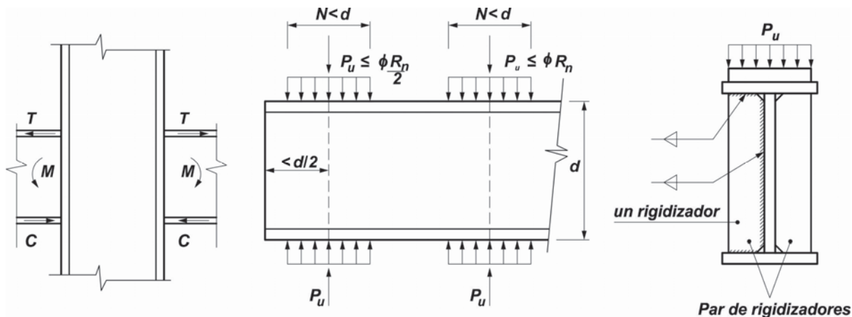
Figura J.10.4. Pandeo por compresión del alma.
