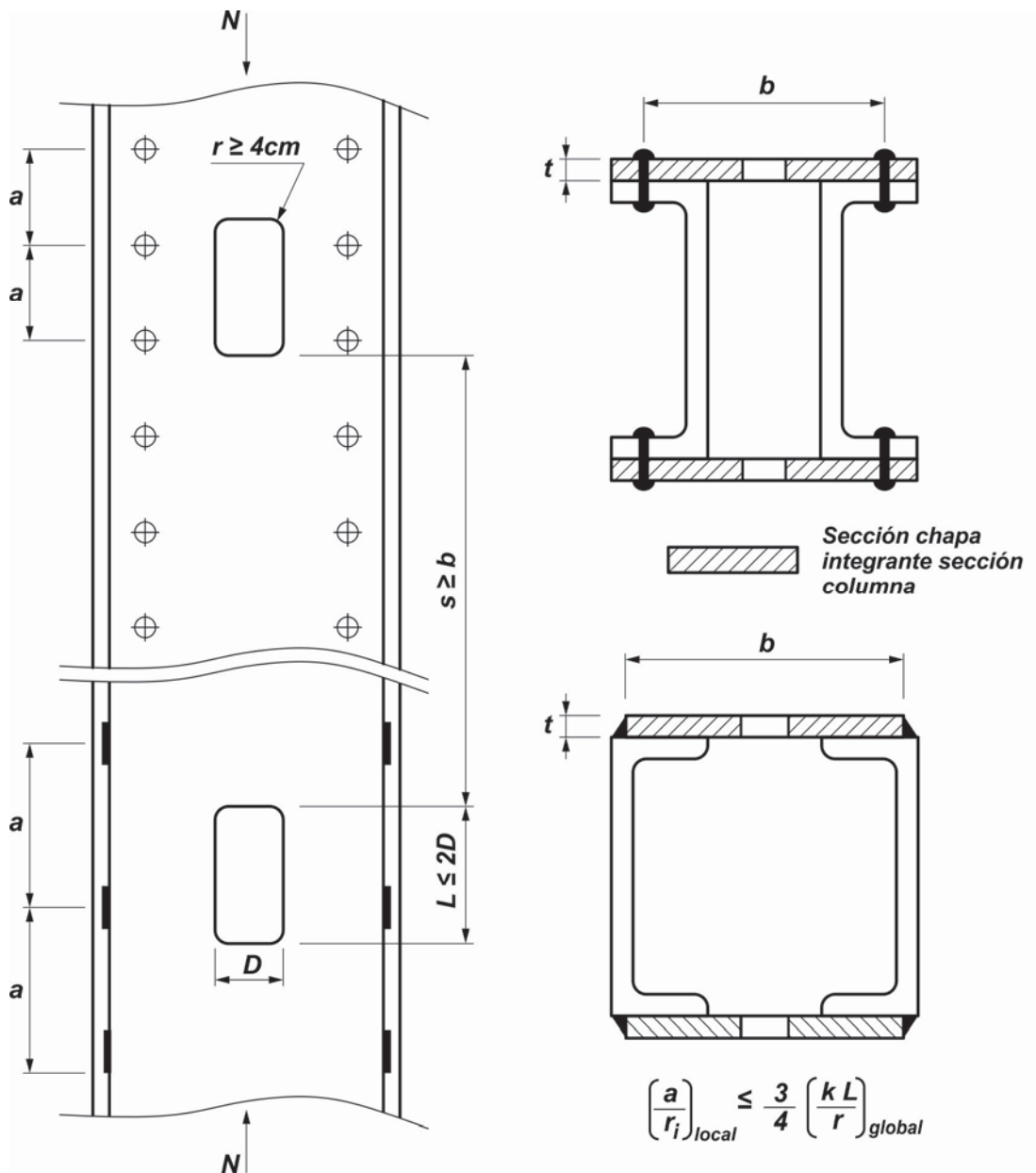
Figura E.6.5. Barras armadas del Grupo III.
