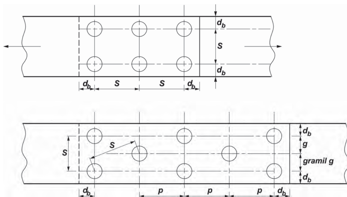
Figura J.3.1. Separación entre centros de agujeros.
