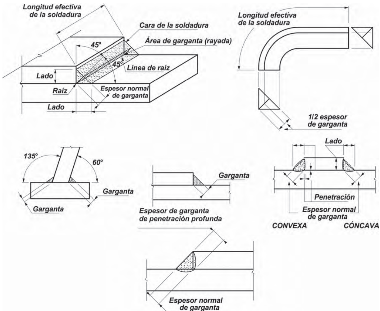
Figura J.2.3. Nomenclatura de soldaduras de filete.
