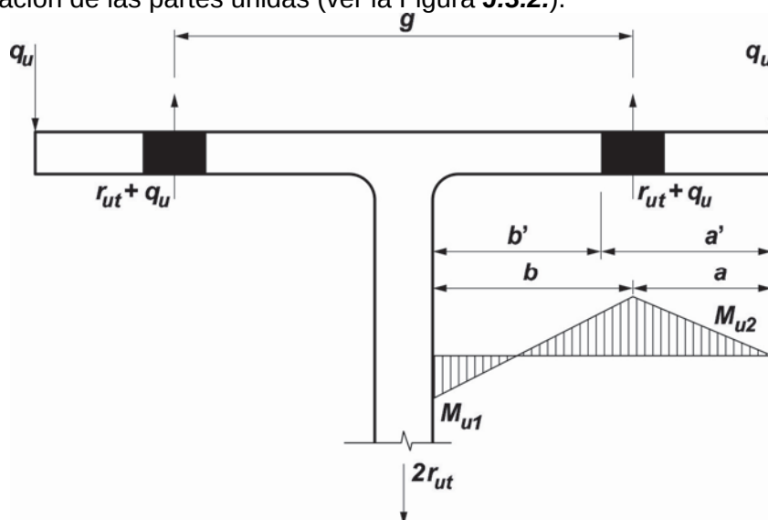
Figura J.3.2. Acción de palanca.
