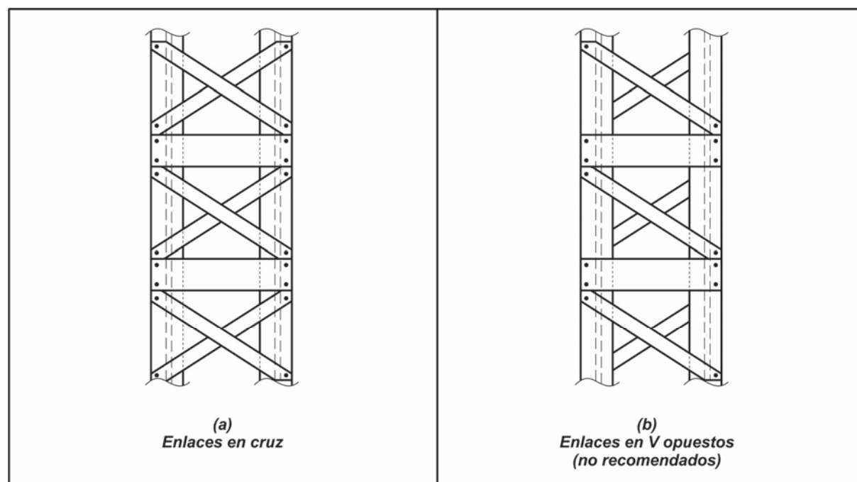
Figura E.6.10. Celosías combinadas con presillas.
