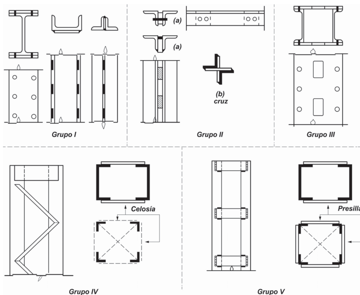
Figura E.6.1. Barras armadas comprimidas.
