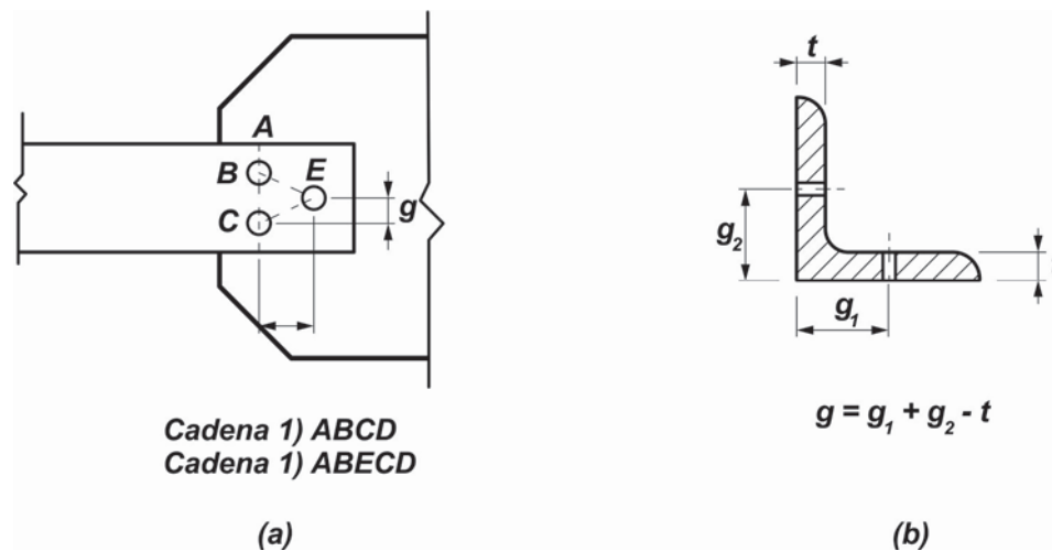
Figura B.4.3. Áreas netas.
