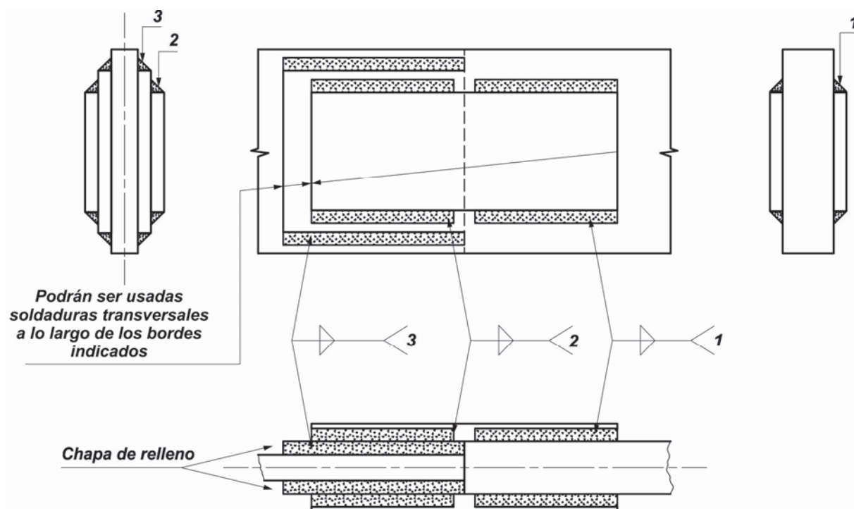
Figura J.5.2. Chapa de relleno con espesor mayor o igual que 6 mm.
