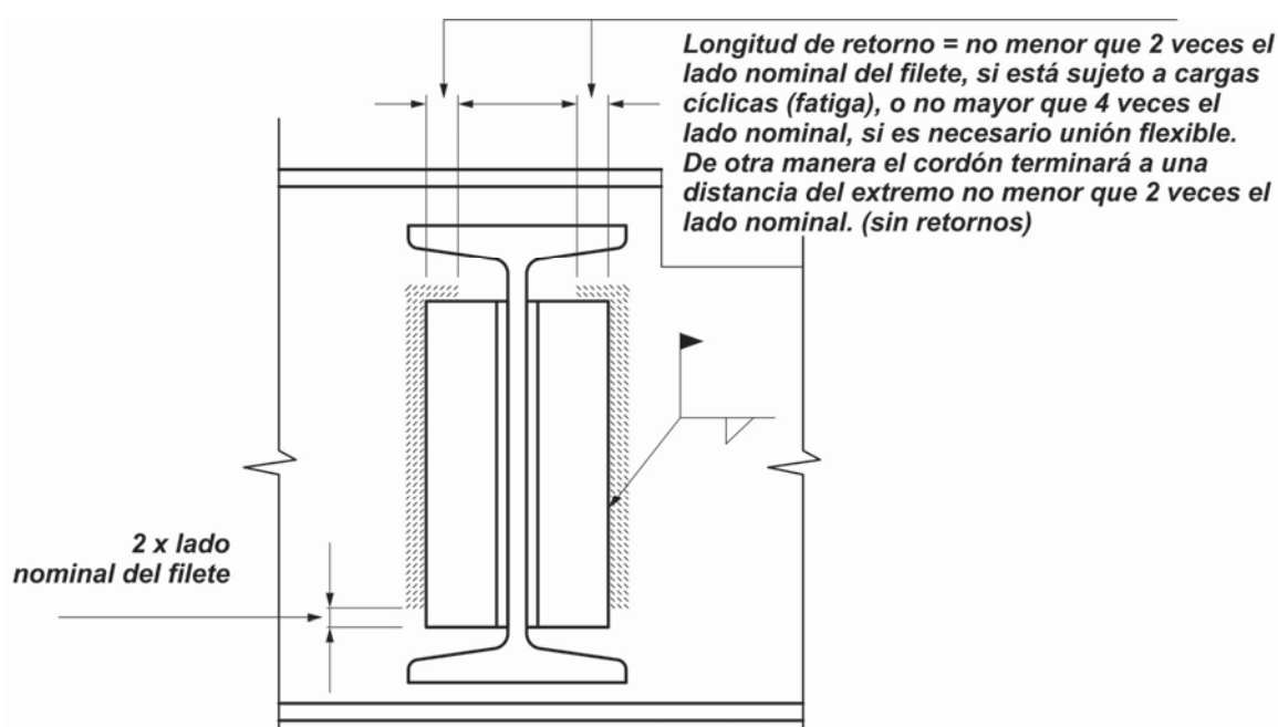
Figura J.2.5. Retornos.
