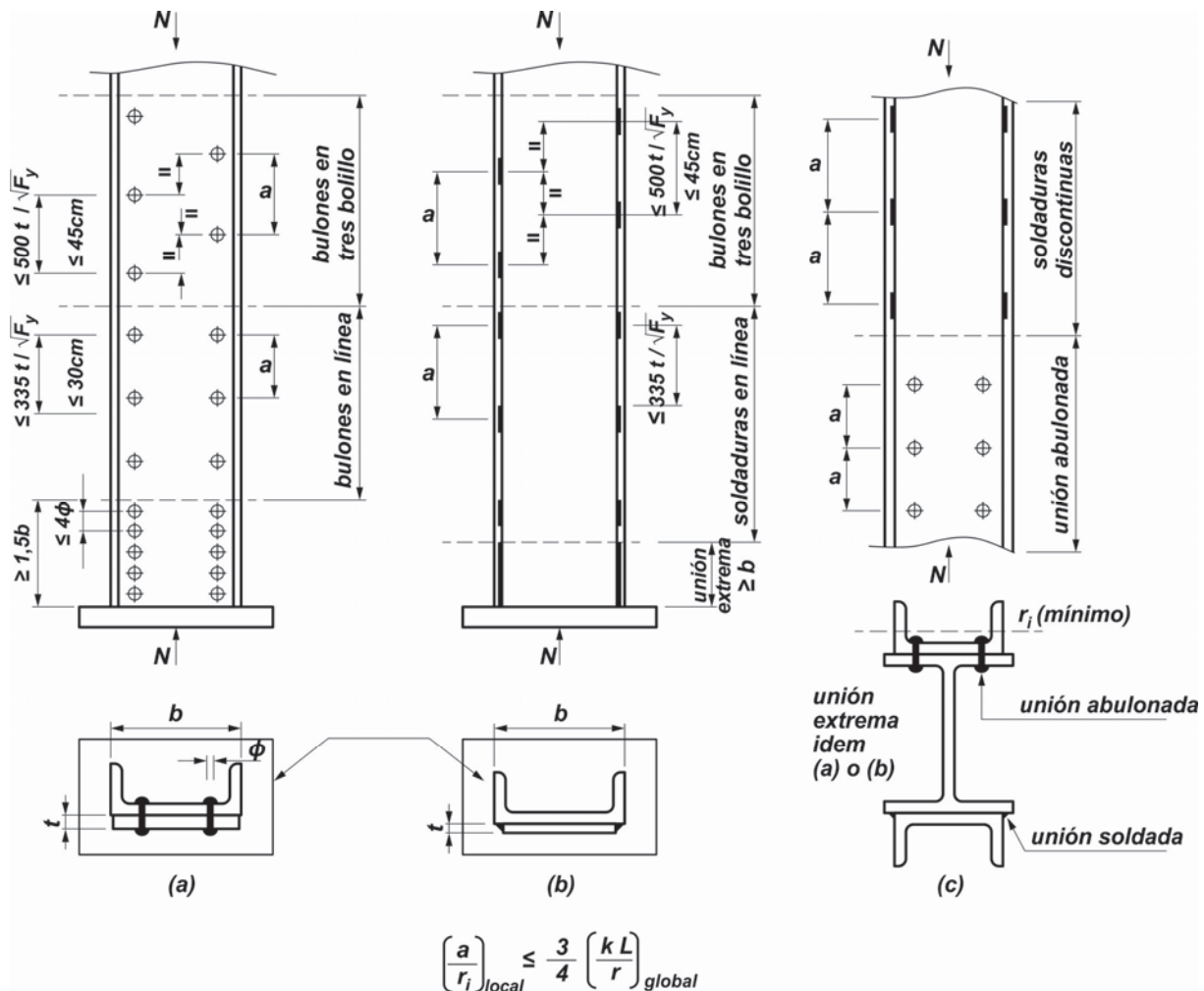
Figura E.6.3. Barras armadas del Grupo I.
