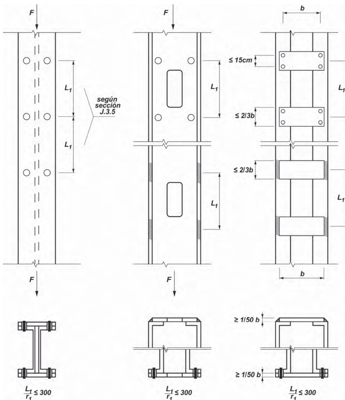
Figura D.4.1. Barras armadas traccionadas.
