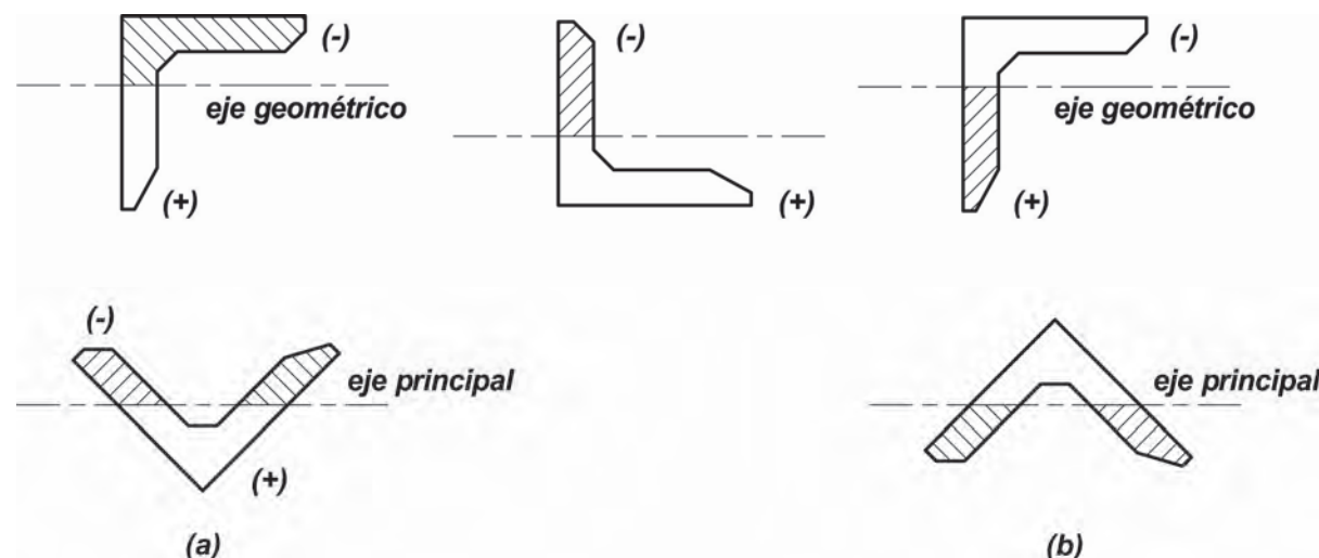
Figura F.10.1. Solicitaciones en punta de ala.
