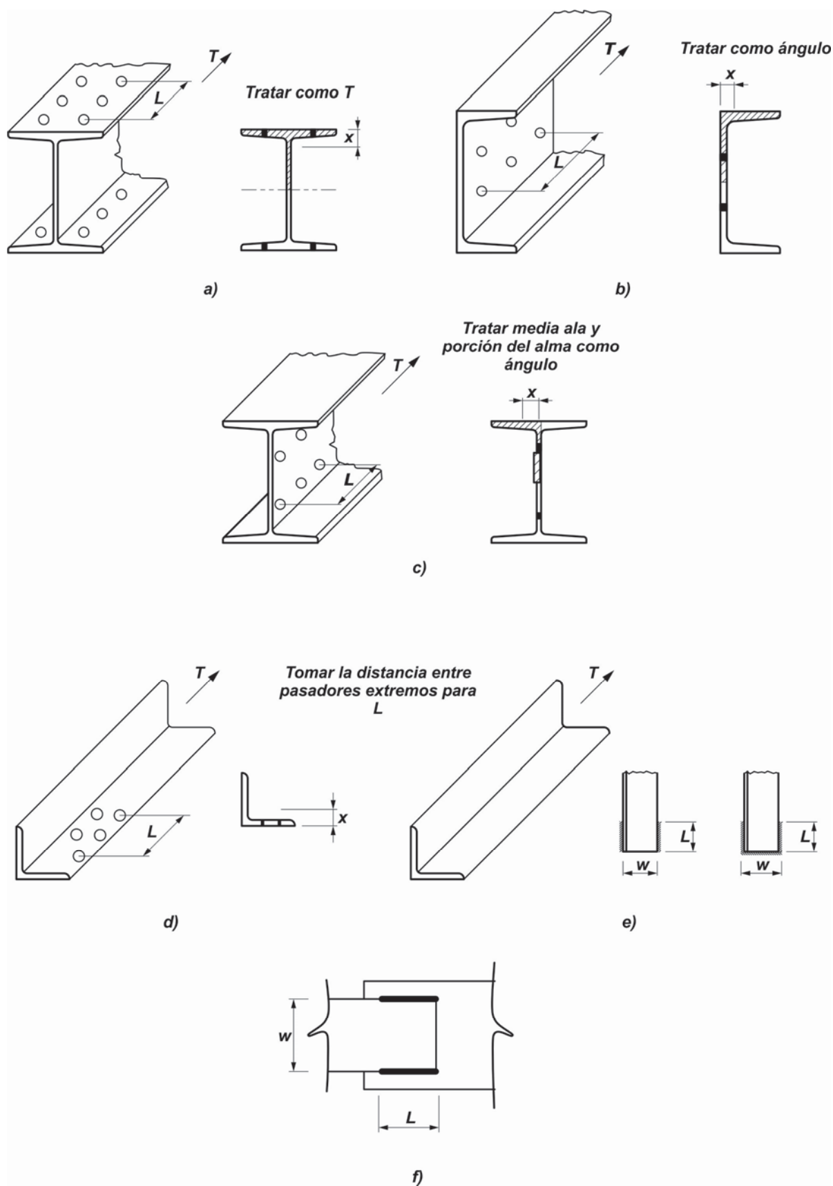
Figura D.3.1. Determinación de \bar{x} y L .
