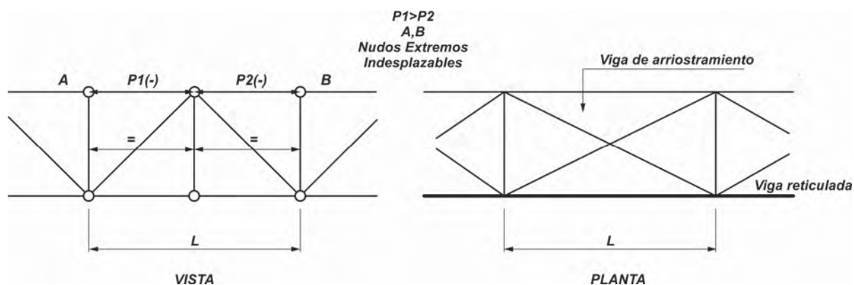
Figura 7.2.1. Cordones con distinta carga axil.
