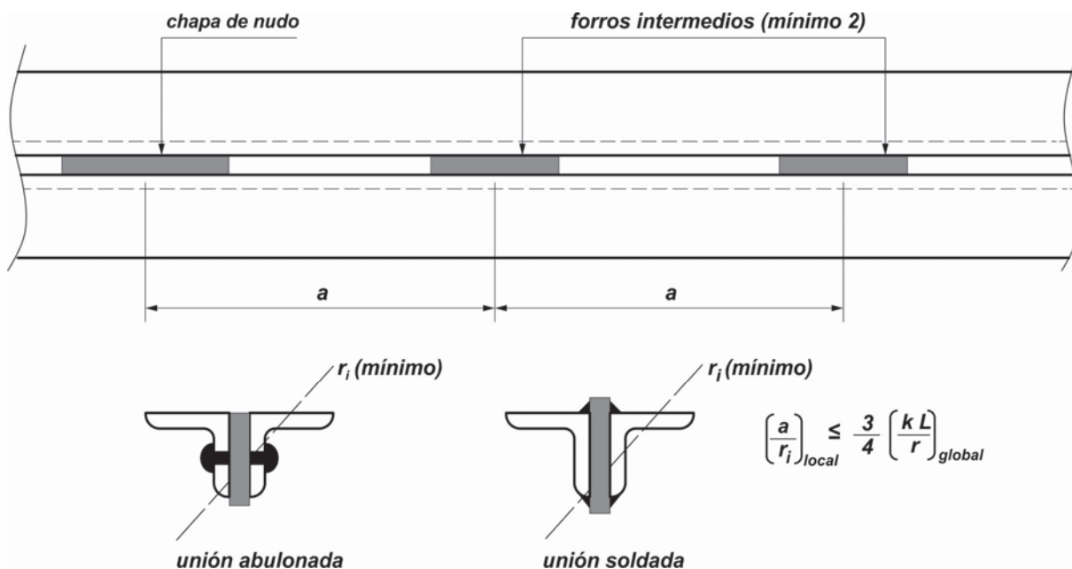
Figura E.6.4. Barras armadas del Grupo II.
