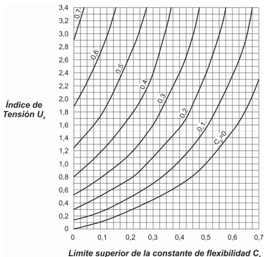
Figura 2.2. Coeficiente de flexibilidad límite para sistemas secundarios.
