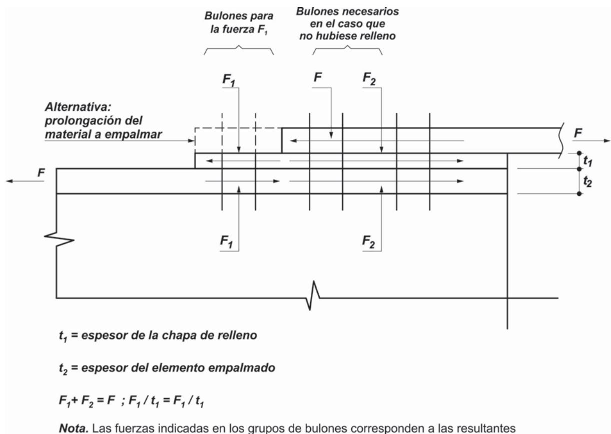
Figura J.5.3. Chapas de relleno en uniones abulonadas.
