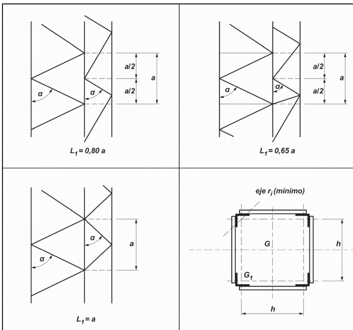
Figura E.6.7. Determinación de L_1 .
