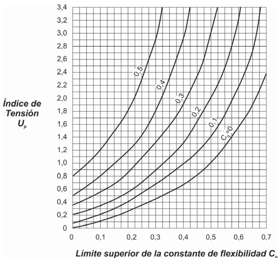
Figura 2.1. Coeficiente de flexibilidad límite para sistemas primarios.
