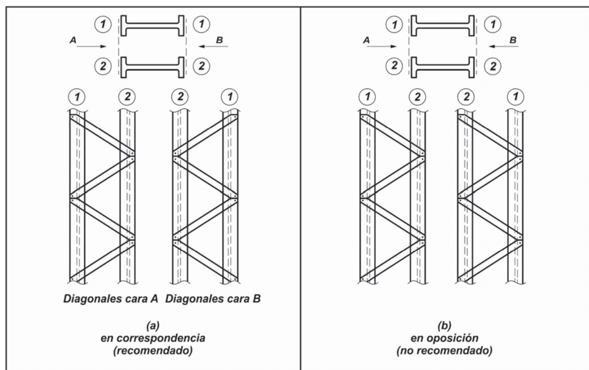
Figura E.6.9. Triangulaciones simples.
