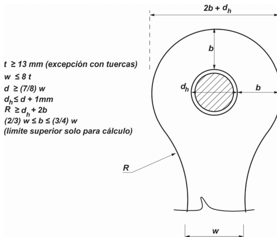
Figura D.6.1. Especificaciones dimensionales. Barras de ojo.
