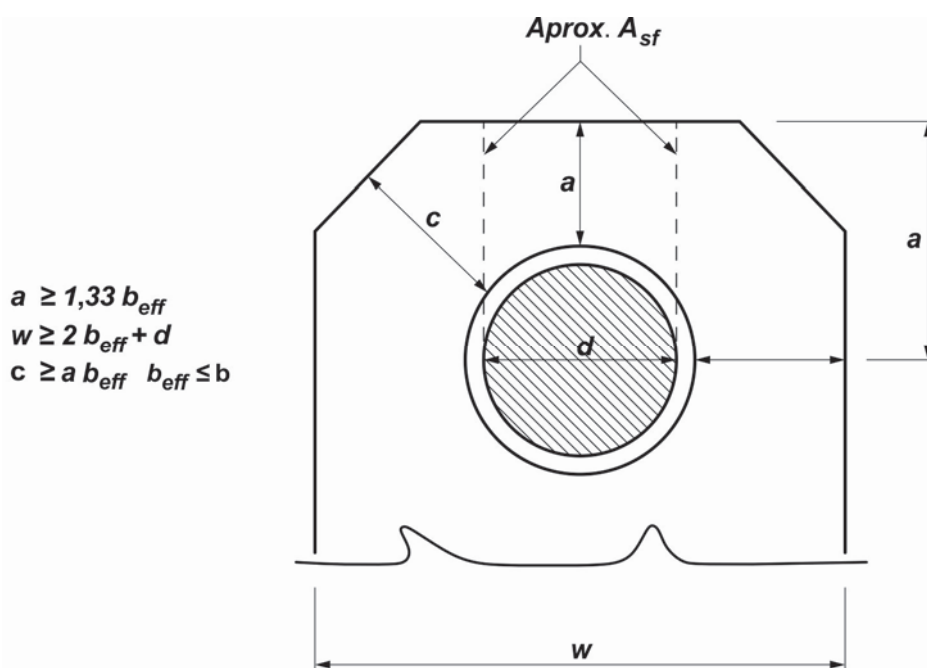
Figura D.5.1. Especificaciones dimensionales. Barras unidas por pernos.
