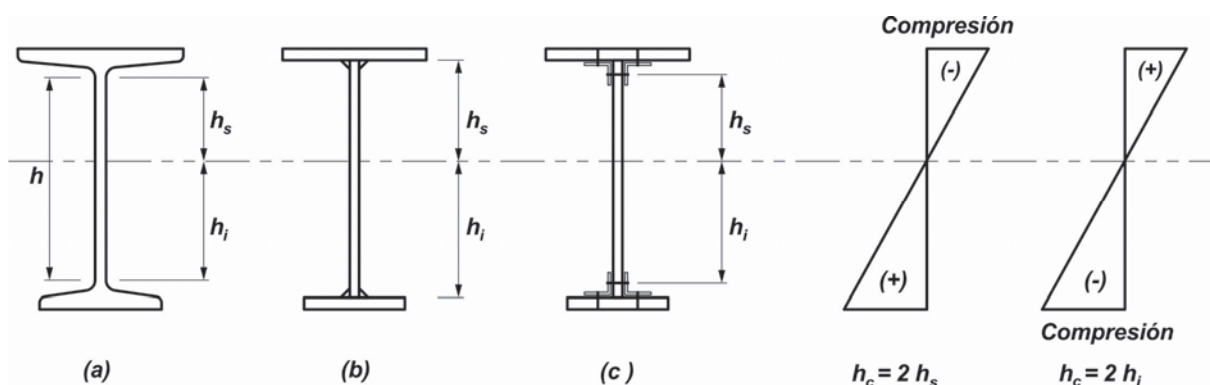
Figura B.4.1. Determinación de h_c .
