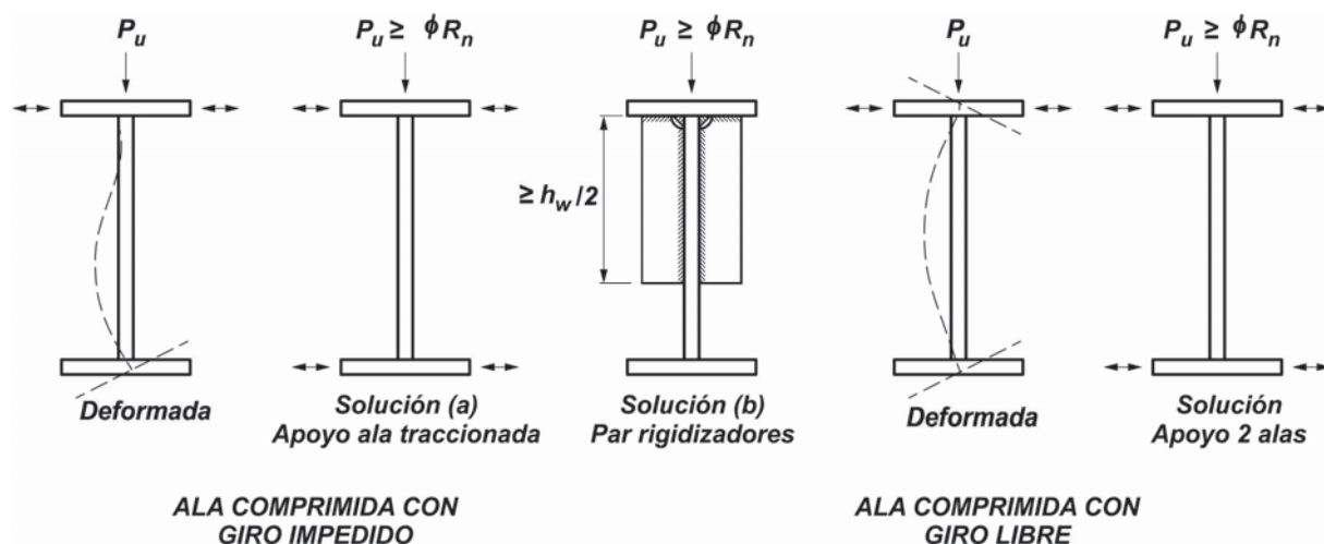
Figura J.10.3. Pandeo lateral del alma.
