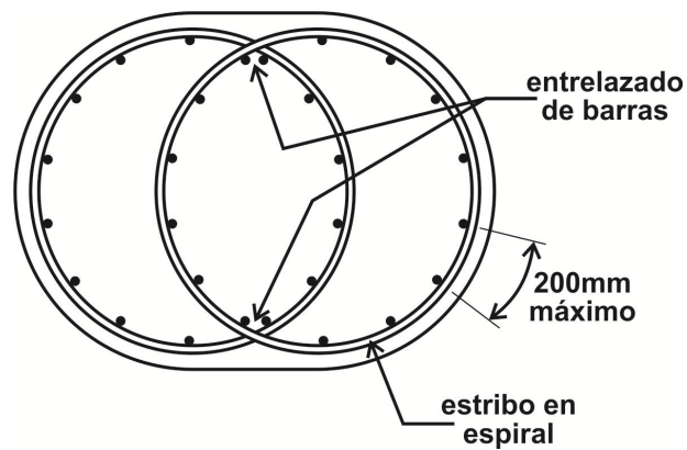
Figura C5.10.11.4.1d-3: Detalles de Entrelazado de Estribos en Columnas
