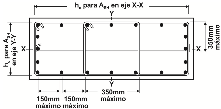
Figura C5.10.11.4.1d-4: Detalles de Estribos en Columnas
