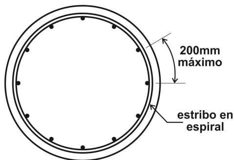
Figura C5.10.11.4.1d-1: Columna con armadura transversal de espiral simple
