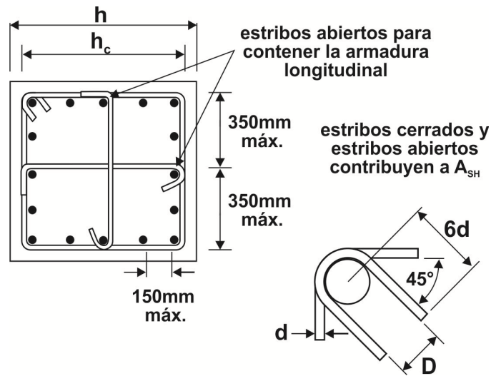
Figura C5.10.11.4.1d-2: Detalles de Estribos en Columnas
