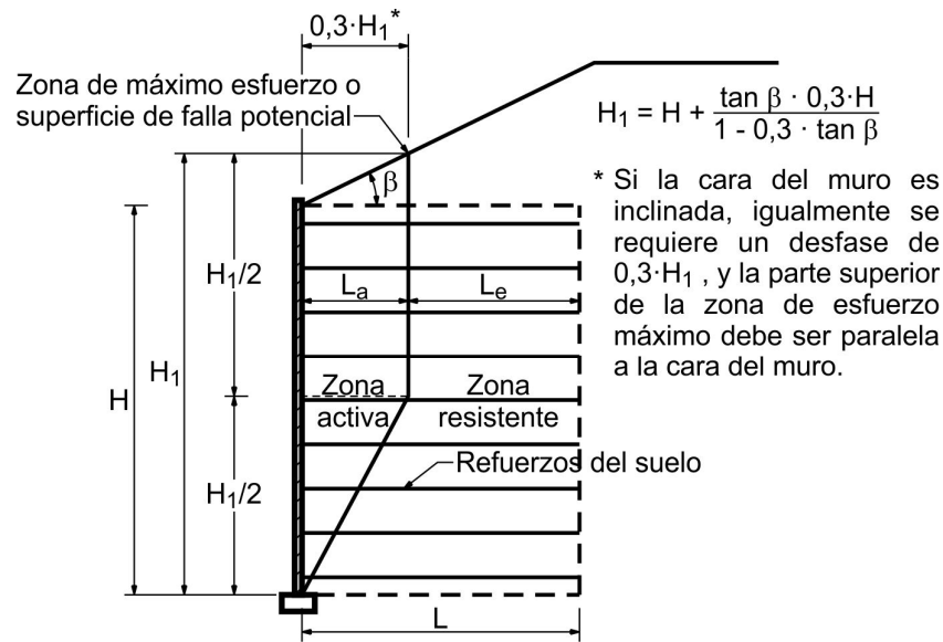
(a) Refuerzos inextensibles
