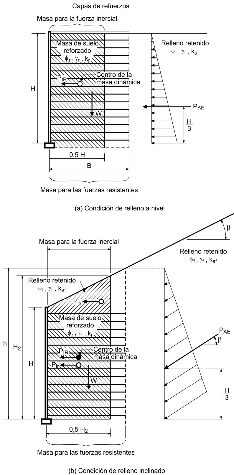
Figura 11.10.7.1-1. Estabilidad externa de un muro de suelo estabilizado mecánicamente sujeto a carga sísmica
