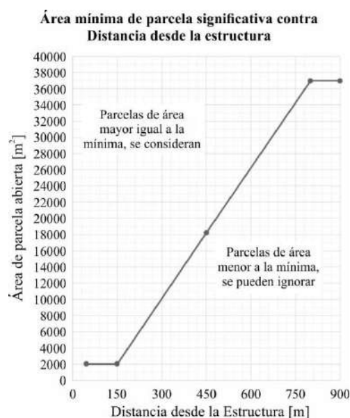
Figura C 1.7-4. Área mínima de parcelas abiertas individuales que afecta la Calificación de la Exposición B.
