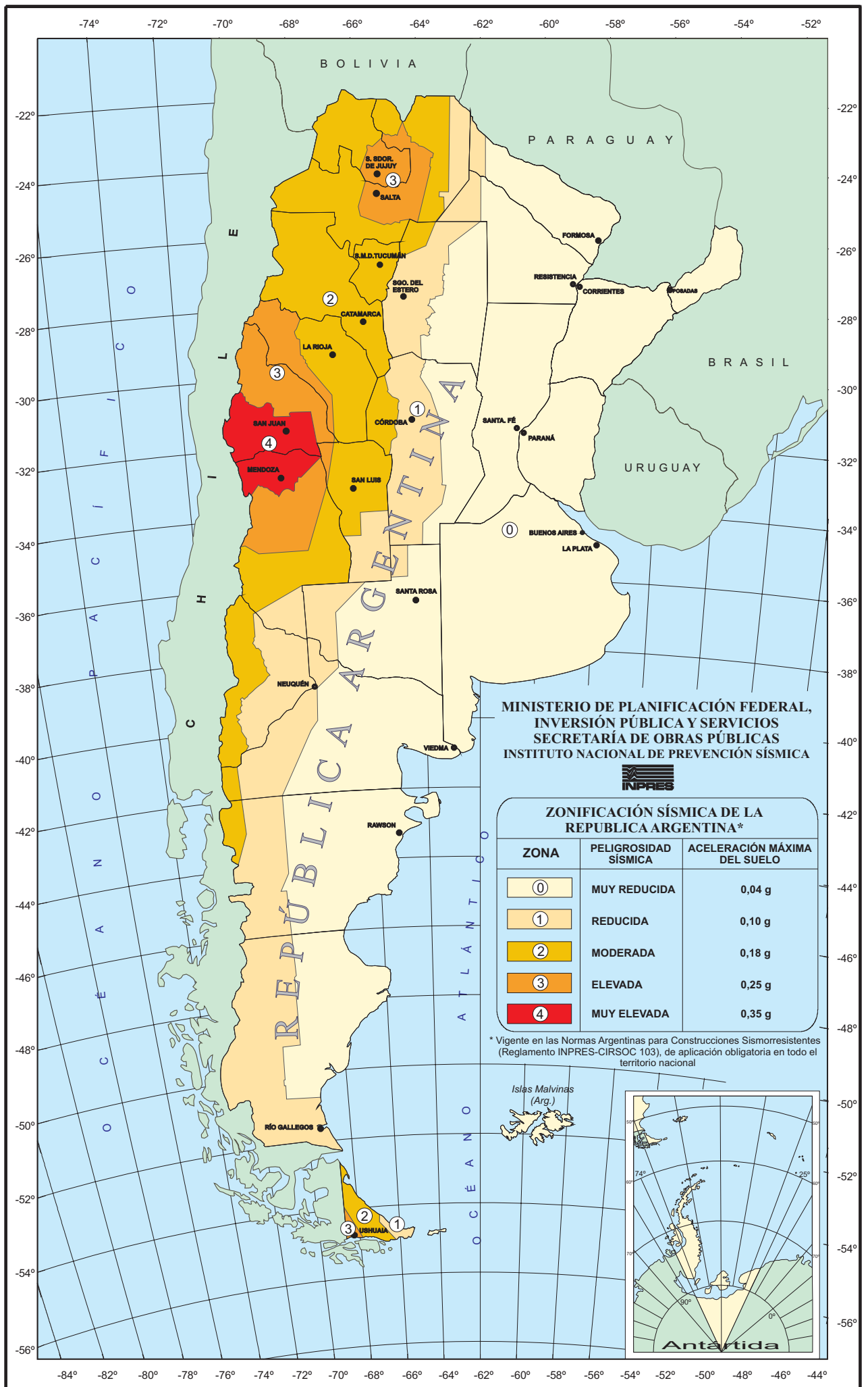
Mapa de Zonificación sísmica de la República Argentina
