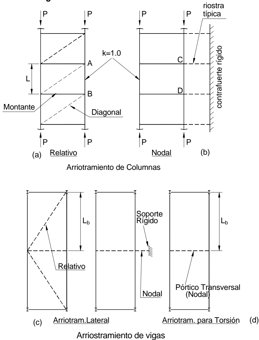
Figura C-A.6-1. Tipos de sistemas de arriostramiento
