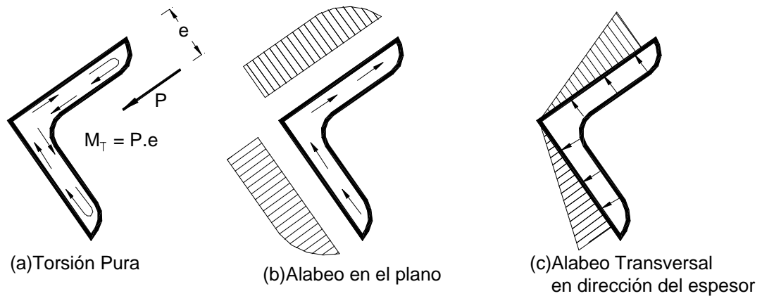
Figura C-G.4-1. Tensiones tangenciales debidas a torsión
