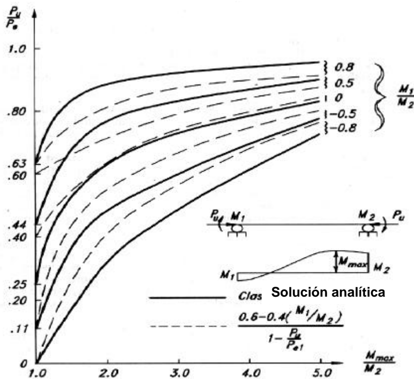
Figura C-A.8-4. Momentos de Segundo Orden máximos para vigas columnas solicitadas por momentos en los extremos
