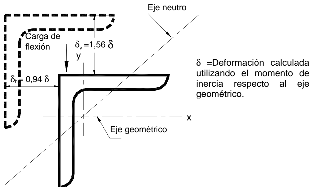
Figura C-F.10-2. Flexión alrededor de un eje geométrico de ángulo de alas iguales lateralmente no arriostrado.
