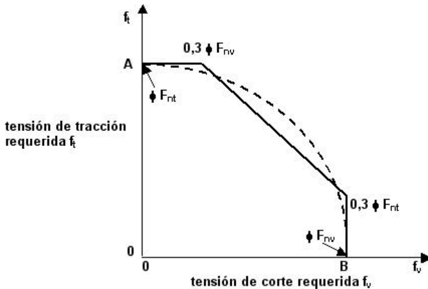
Figura C-J.3-6. Aproximación trilineal para solución elíptica
