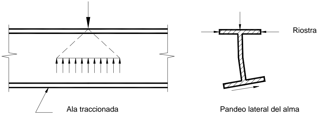
Figura C-J.10-3. Pandeo lateral del alma
