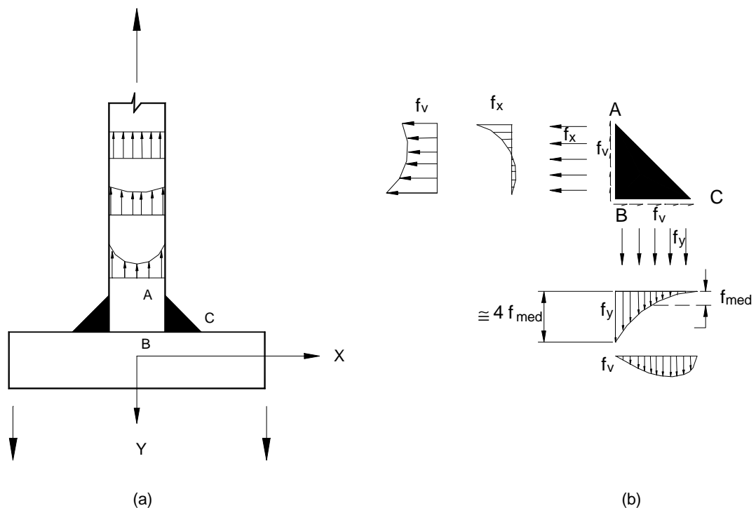
Figura C-J.2-15. Distribución de tensiones en una junta en T con cordones de filete (corte transversal al filete)
