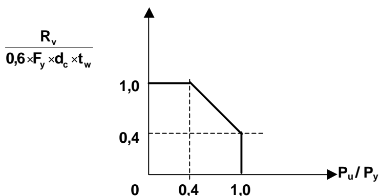
Figura C-J.10-6. Interacción de corte y fuerza axil (elástica)
