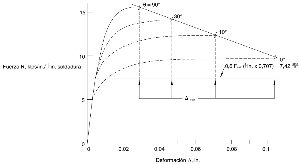
Figura C-J.2-16. Relación Carga-Deformación de un cordón de soldadura
