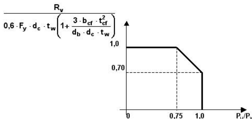
Figura C-J.10-7. Interacción de corte y fuerza axil (inelástica)
