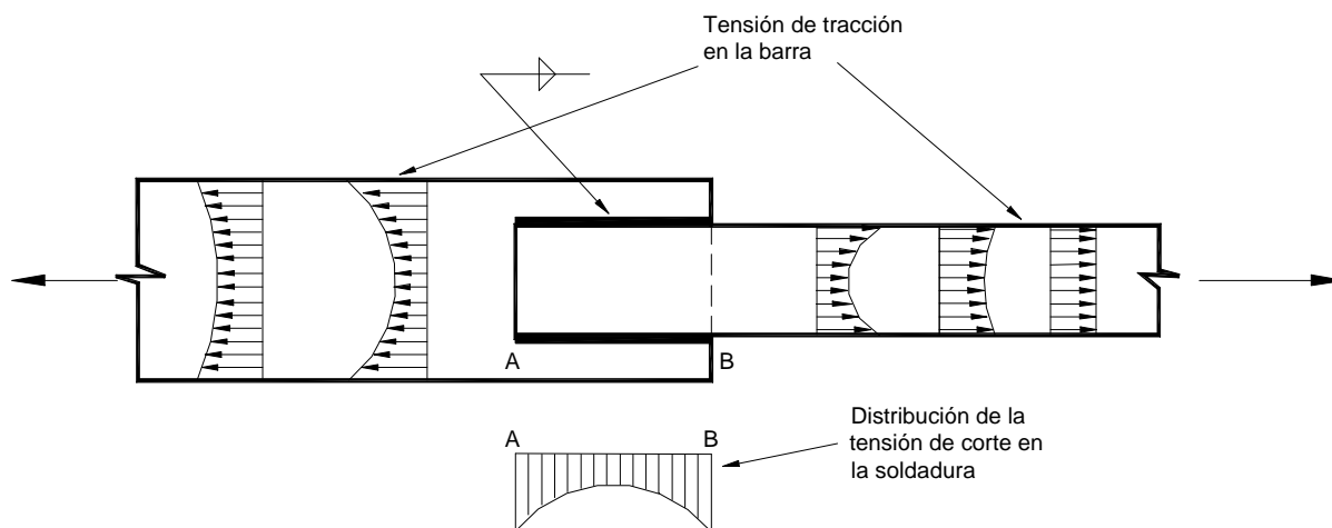
Figura C-J.2-13. Distribución de tensiones en una junta traslapada con cordones de filete longitudinales
