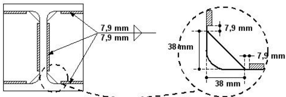
Figura C-J.10-9. Ubicación recomendada para soldaduras de filete de rigidizadores para evitar la zona k
