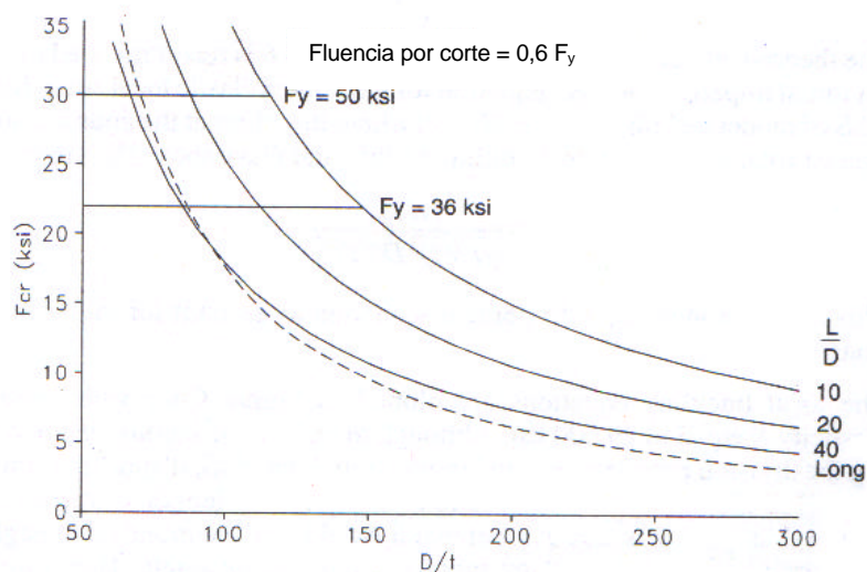
Figura C-H.3-1. Tensión crítica de torsión F_{cr} para tubos circulares
