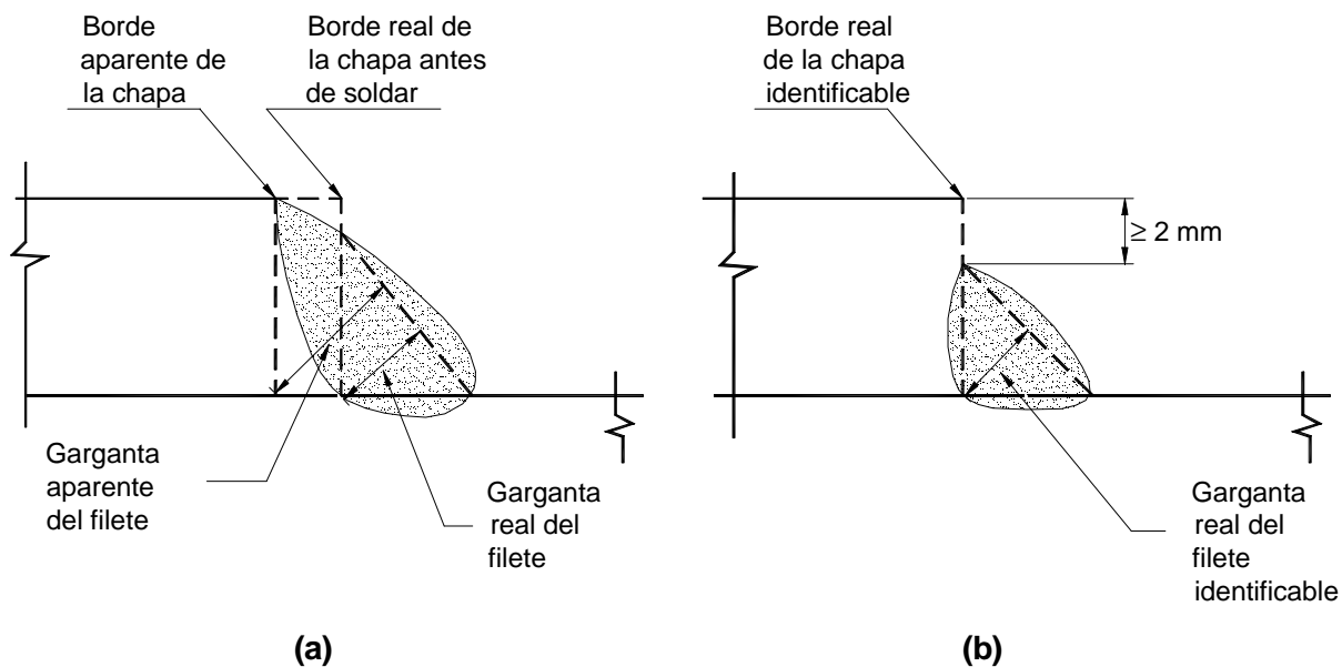
Figura C-J.2-4. Identificación del borde de la chapa
