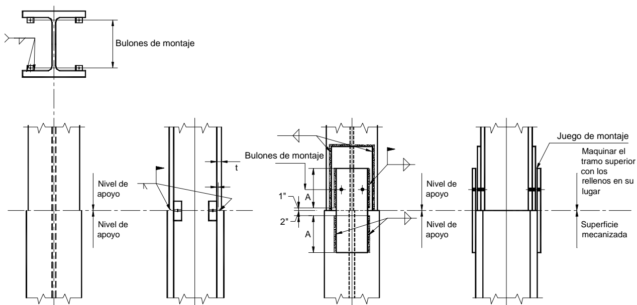
Figura C-J.1-1. Apoyo extremo de columnas por contacto
