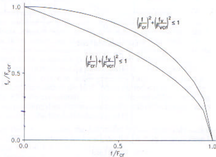
Figura C-H.3-1. Interacción de tensiones normales y tangenciales
