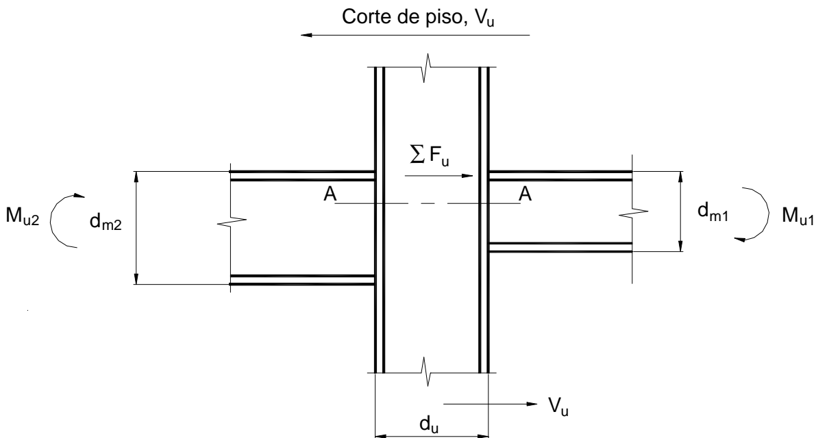
Figura C-J.10-5. Fuerzas de corte en panel nodal
