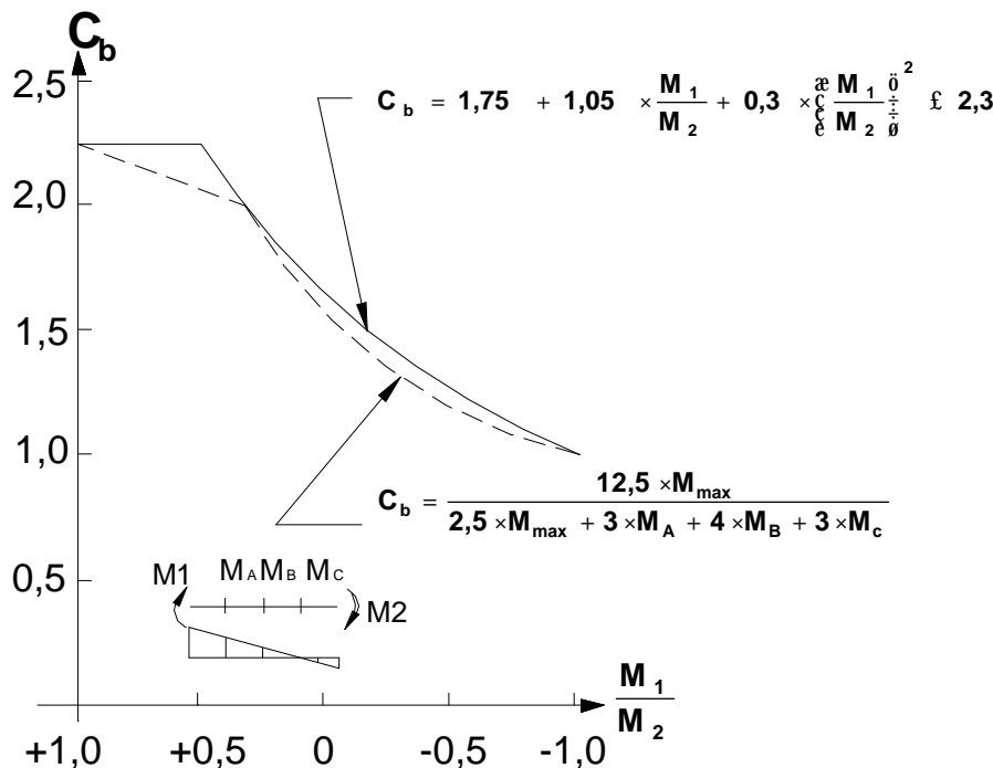
Figura C-F.1-1. Coeficiente C_b en vigas prismáticas para diagramas de momento lineales
