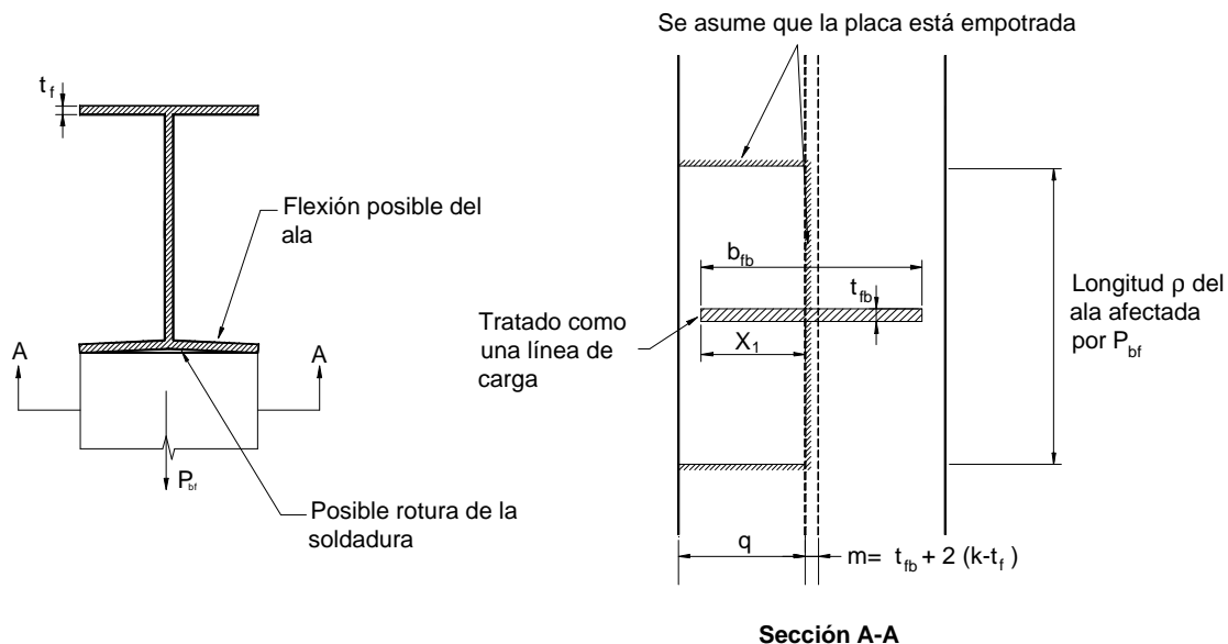
Figura C-J.10-1. Flexión local del ala
