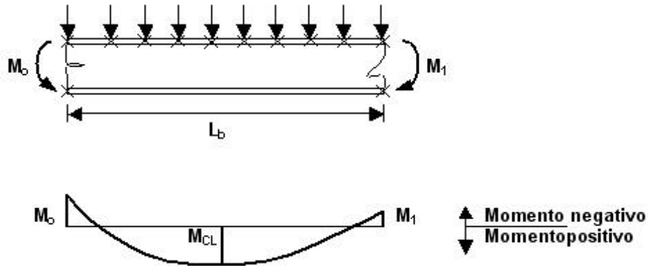
Figura C-F.1-2. Convención de signos de momentos para fórmula (C-F.1-5)
