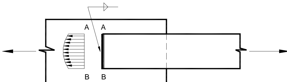
Figura C-J.2-14. Distribución de tensiones en una junta traslapada con cordones de filete transversales
