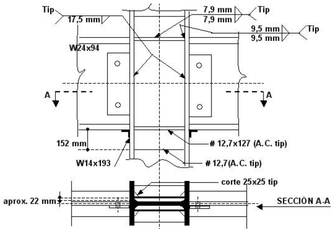
Figura C-J.10-10. Ejemplo de rigidizador y chapa de refuerzo con soldadura de filete
