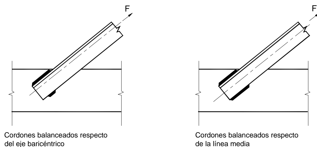
Figura C-J.1-4. Soldaduras balanceadas para miembros sometidos a cargas cíclicas
