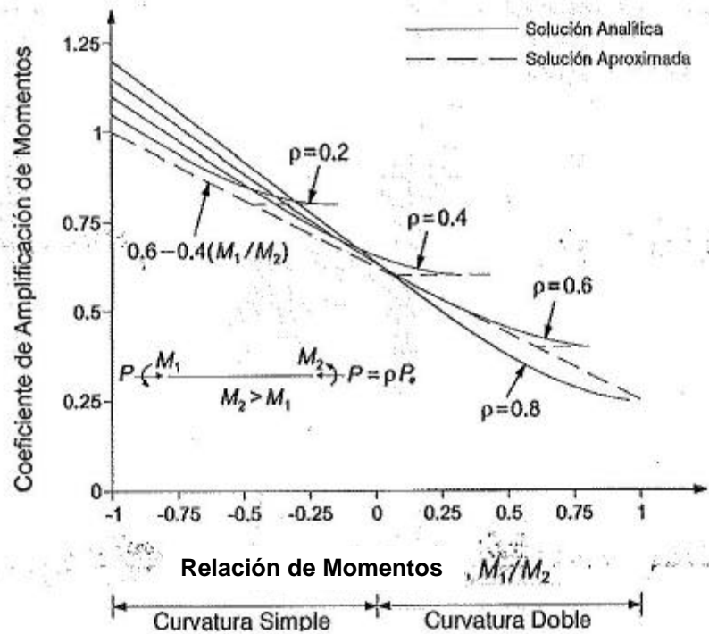
Figura C-A.8-3. Factor C_m para momentos equivalentes de vigas-columnas solicitadas por momentos en los extremos
