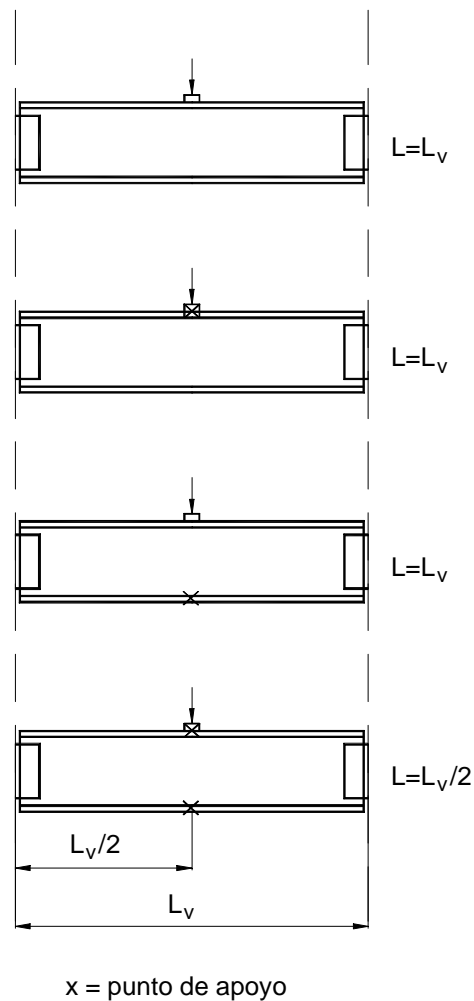
Figura C-J.10-4. Longitud de ala lateralmente arriostrada
