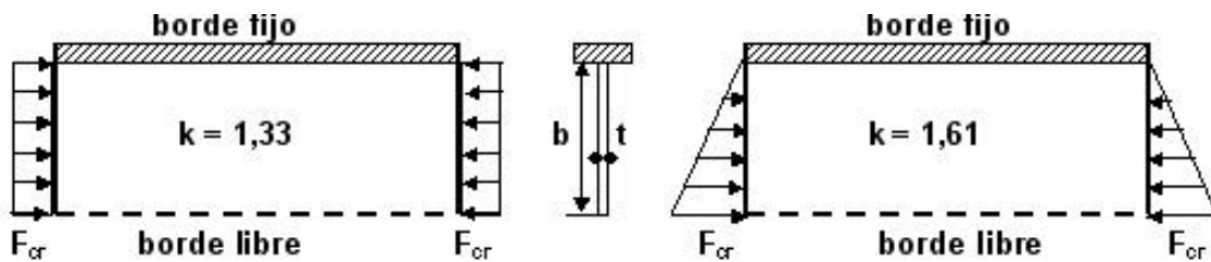
Figura C-F.9-1. Coeficientes de abolladura para compresión uniforme y compresión linealmente variable
