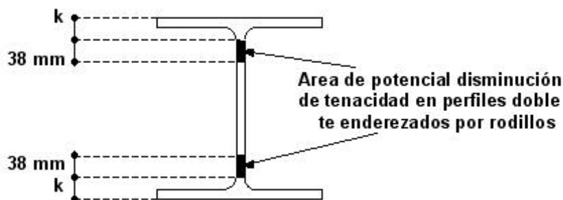
Figura C-J.10-8. Zona k representativa de un perfil de ala ancha
