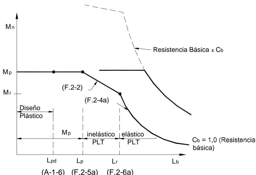
Figura C-F.2-1. Momento nominal en función de la longitud lateralmente no arriostrada y del diagrama de momento
