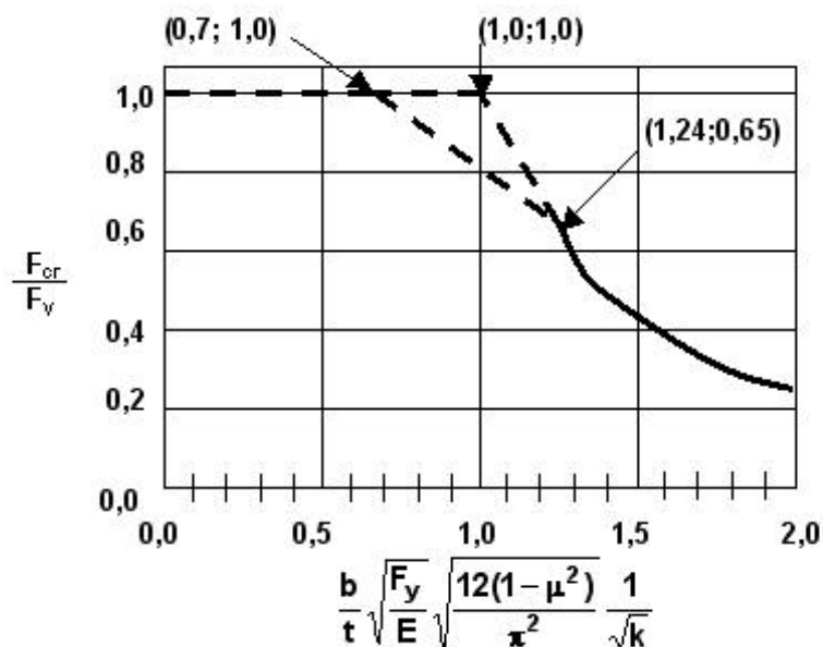
Figura C-F.9-2. Esquema general de las tensiones críticas de pandeo en placas
