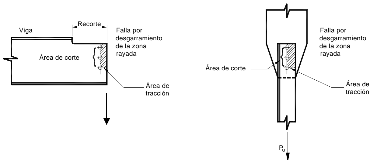
Figura C-J.4-1. Superficie de falla para el estado límite de rotura de bloque de corte
