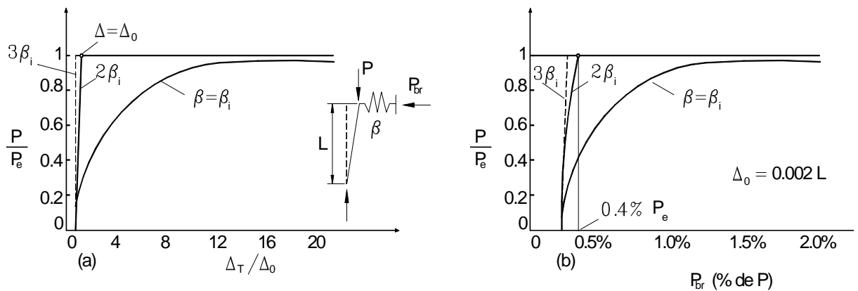
Figura C-A-6-3. Efectos del desplazamiento inicial fuera del plano
