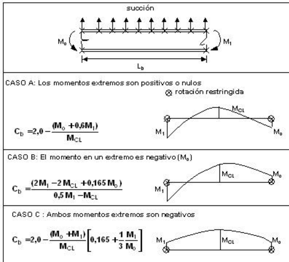
Figura C-F.1-4. Factores C_b para cargas de succión en vigas con ala superior con arriostramiento continuo
