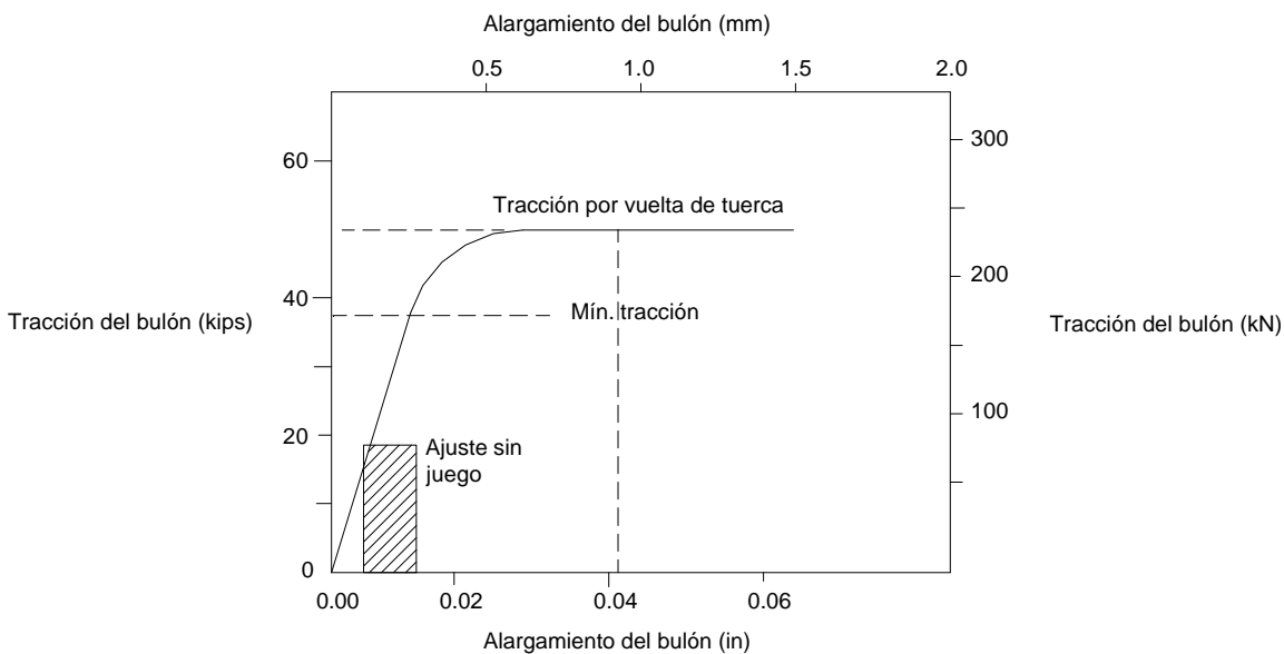
Figura C-J.3-4. Relación carga-alargamiento de un bulón
