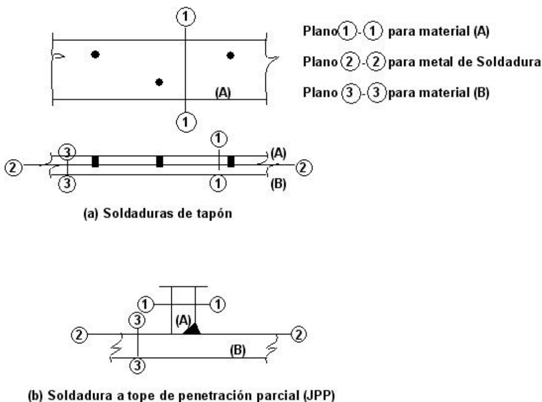
Figura C-J.2-12. Planos de corte para soldaduras de tapón y a tope de penetración parcial
