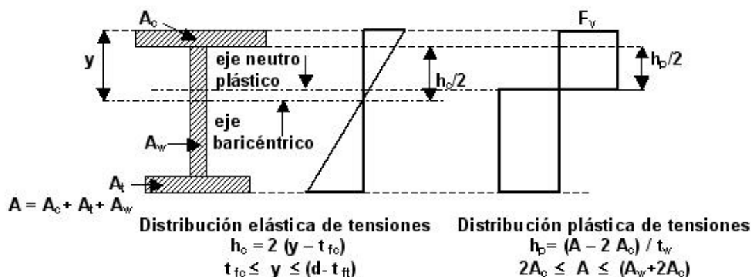
Figura C-F.4-1. Distribución de tensiones elásticas y plásticas
