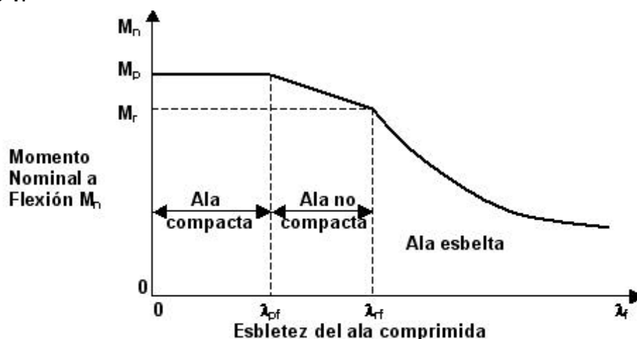
Figura C-F.3-1. Resistencia Nominal a flexión en función de la esbeltez del ala comprimida
