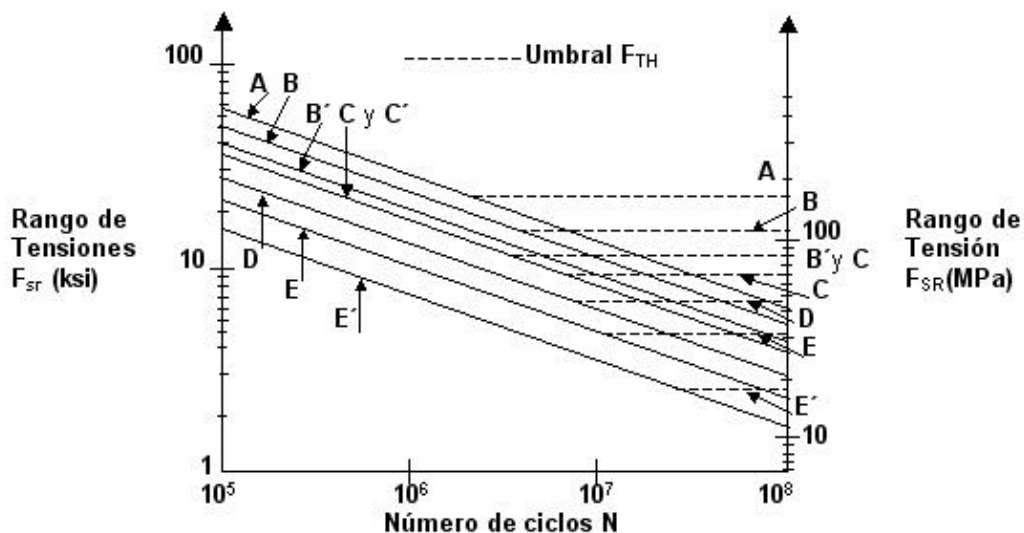
Figura C-A.3-1. Curvas de resistencia a la fatiga
