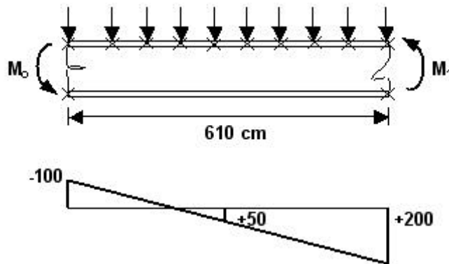
Figura C-F.1-3. Diagrama de momentos para el ejemplo de aplicación de la fórmula (C-F.1-5)
