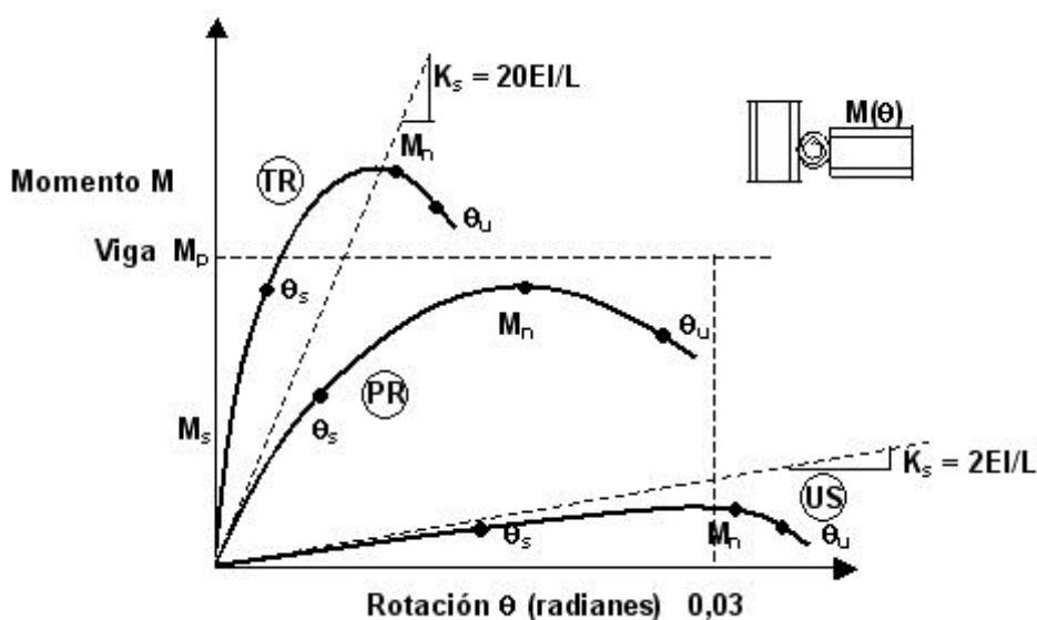
Figura C-B.3-4. Clasificación de curvas de respuesta momento-rotación de uniones totalmente restringidas (TR), parcialmente restringidas (PR) y uniones Simples (US)
