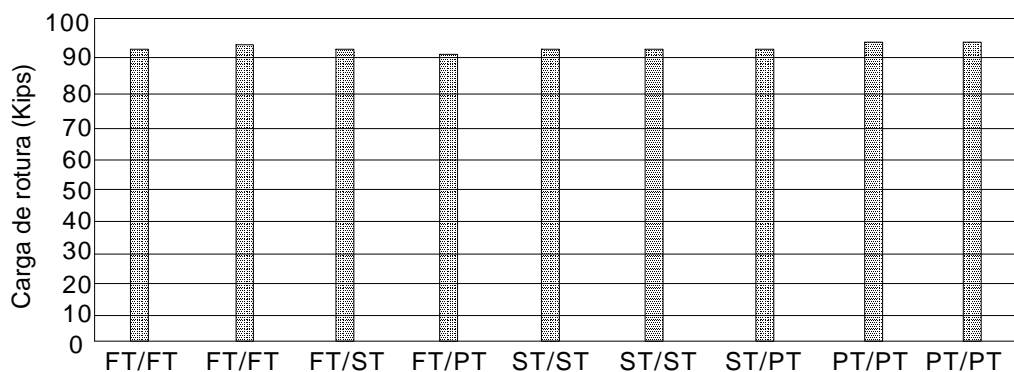
Figura C-J.3-2. Ensayos de Johnson (1996) Bulones ASTM A325 diámetro 3/4", longitud 2 3/4"(70 mm)
