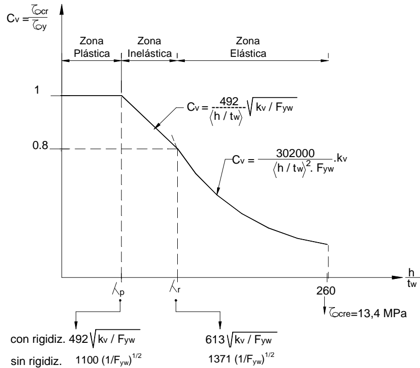
Figura C-G.2-1 (Variación de C_v en función de la relación de esbeltez del alma para E = 200\,000\text{ MPa} )
