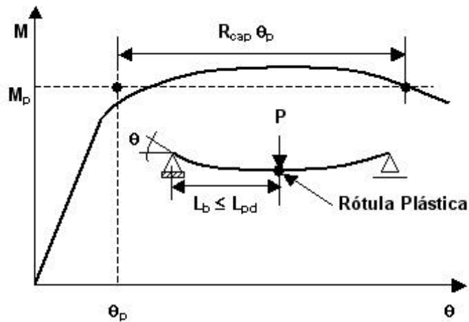
Figura C-A.1-1. Definición de capacidad de rotación
