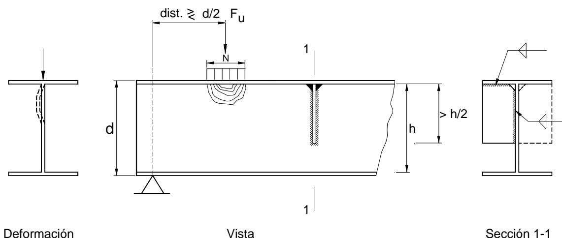
Figura C-J.10-2. Pandeo localizado del alma
