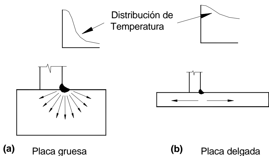
Figura C-J.2-3. Distribución de temperatura en uniones soldadas
