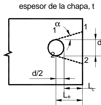
Figura C-J.3-8. Desgarramiento de la chapa
