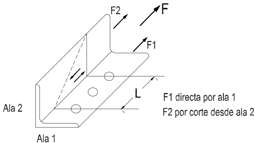
Figura C-D.3-1 Retardo de corte
