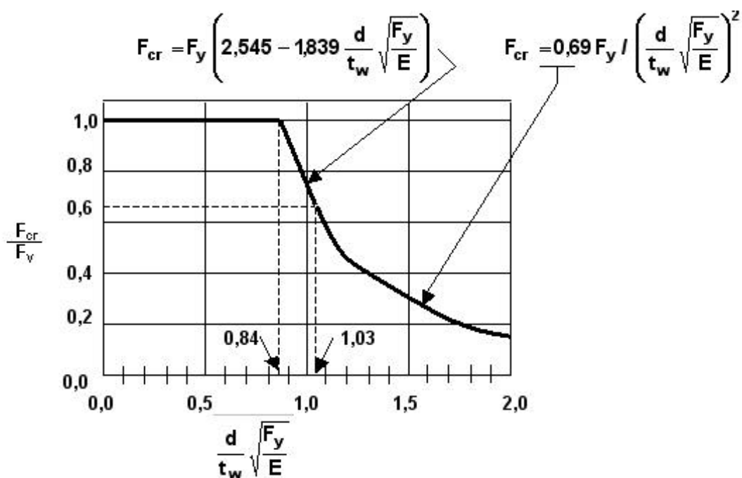
Figura C-F.9-3. Pandeo local del alma de una sección te comprimida por flexión
