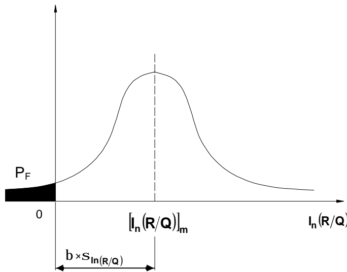
Figura C-B.3-2. Definición del índice de confiabilidad
