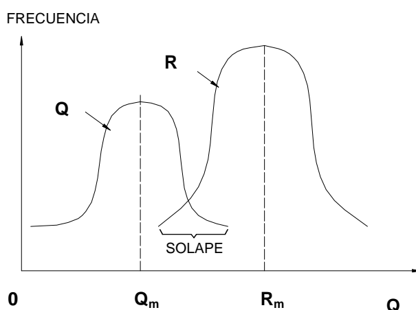
Figura C-B.3-1. Distribución de frecuencias de efectos de las acciones Q y de las resistencias R
