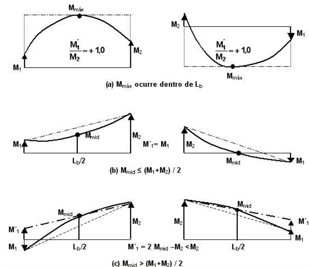
Figura C-A.1-2. Diagramas lineales de momentos equivalentes para calcular M'_1
