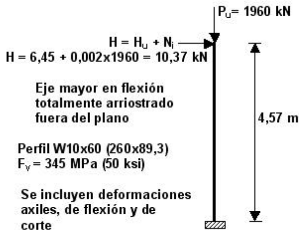
Figura C-C.2-4. Ejemplo de potenciales errores asociados con el uso de un elemento único por miembro en un análisis P-D
