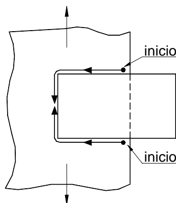
Figura C-J.2-8. Dirección de soldado sugerida para evitar muescas
