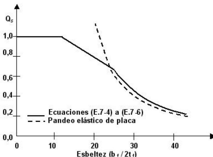
Figura C-E.7-2. Q_s para perfil laminado de ala ancha. F_y = 345 \text{ MPa}
