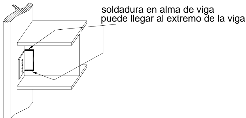
Figura C-J.2-9. Detalle de soldadura de filete en ángulos de unión viga-columna
