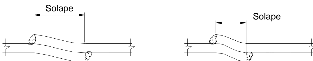
Figura C-J.2-6. Solape Mínimo
