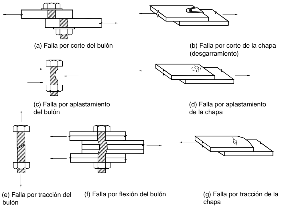
Figura C-J.3-7. Formas posibles de falla en uniones con bulones
