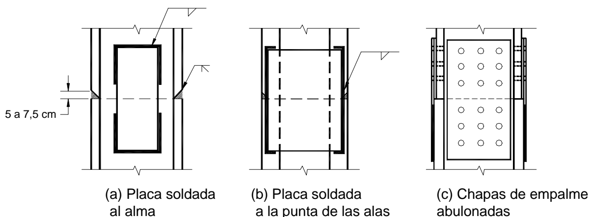
Figura C-J.1-2. Empalmes que minimizan las tensiones por restricción de deformaciones
