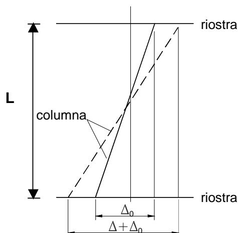
Figura C-C.3-4 . Definiciones
