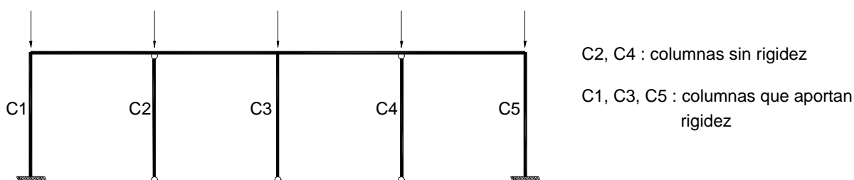
Figura C-A.7.2-3. Pórticos desplazables con columnas sin rigidez lateral
