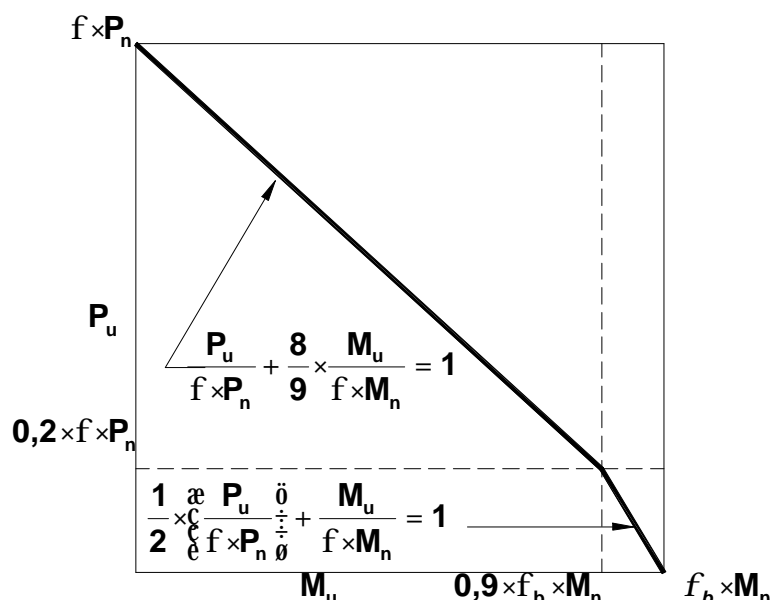
Figura C-H.1-1 Ecuaciones de interacción para vigas-columnas
