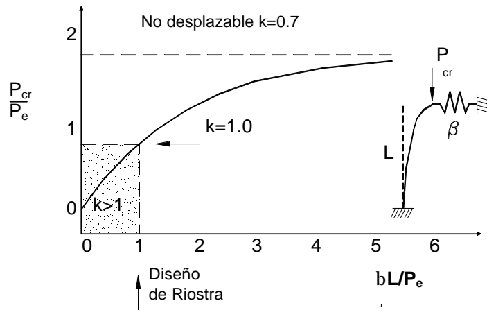
Figura C-A-6-2. Viga en voladizo arriostrada en su extremo libre
