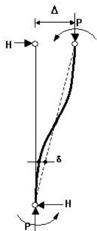
Figura C-C.2-1. Efecto P-D y P-d en vigas-columnas
