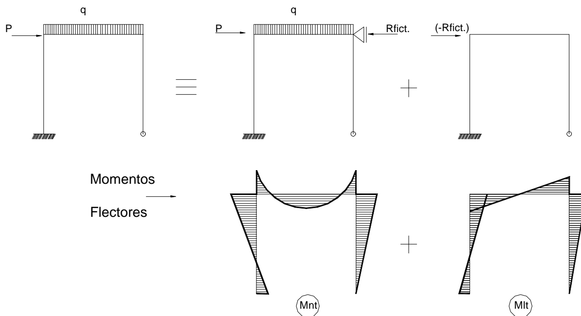
Figura C-A-8-1 Descomposición de momentos flectores
