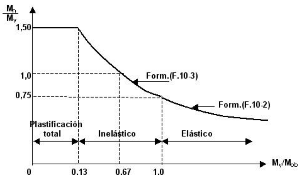
Figura C-F.10-1. Límites para pandeo lateral-torsional de una viga de ángulo simple
