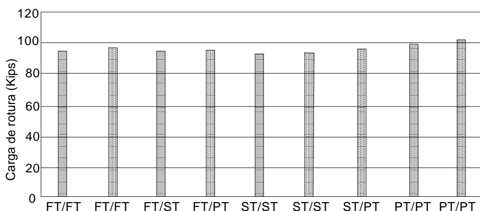
Figura C-J.3-3. Ensayos de Johnson (1996) Bulones ASTM A325 diámetro 3/4", longitud 3 1/4"(83 mm)
