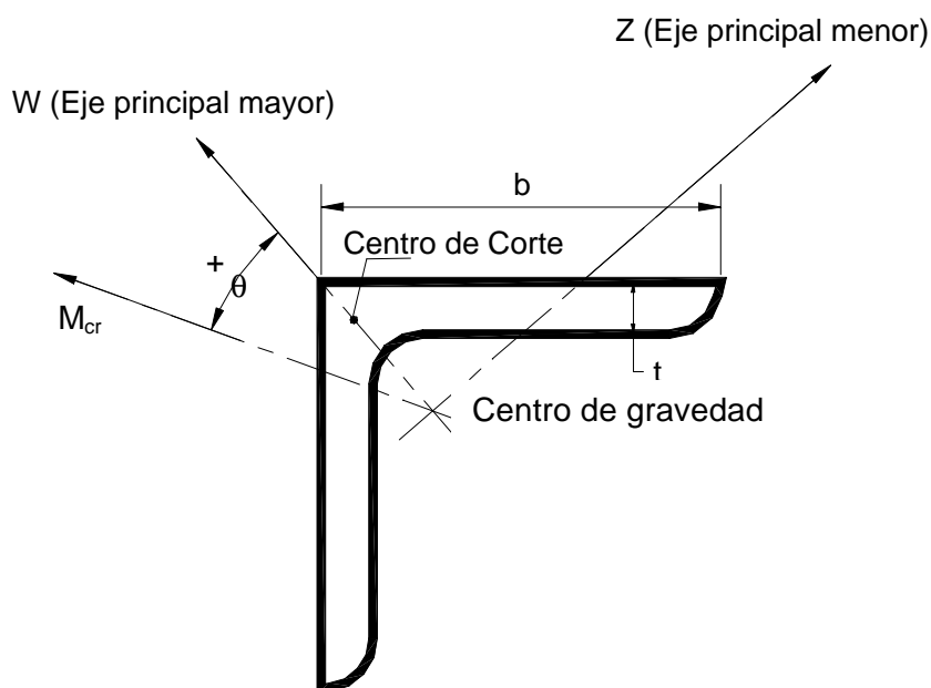
Figura C-F.10-3. Ángulo de alas iguales en caso general de flexión
