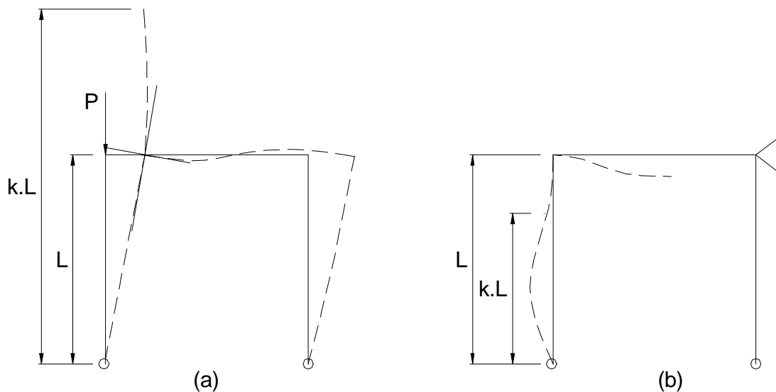
Figura C-A.7.2-1. Longitud efectiva de pandeo de columnas
