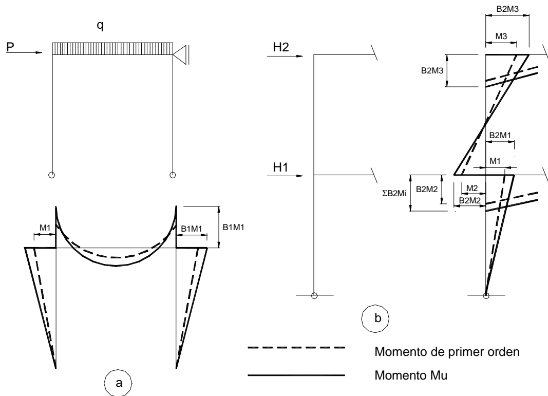
Figura C-A.8-2. Amplificación de momentos
