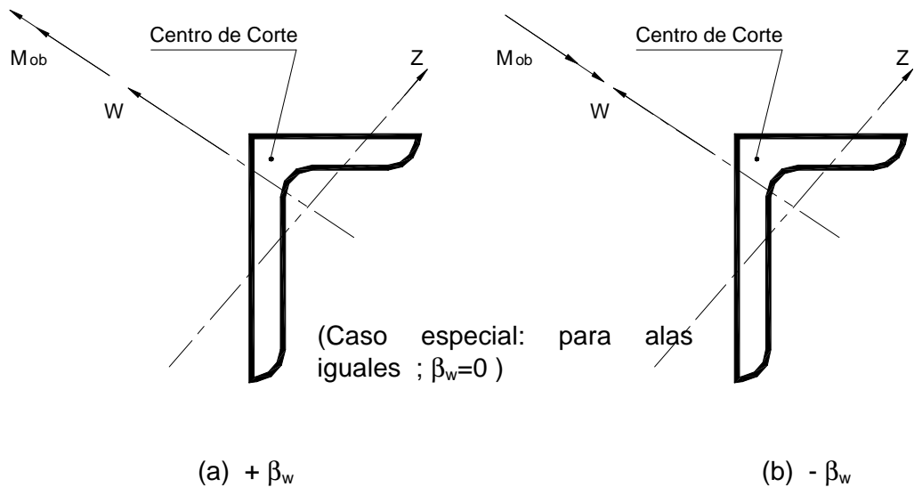
Figura C-F.10-4. Ángulos de alas desiguales en flexión
