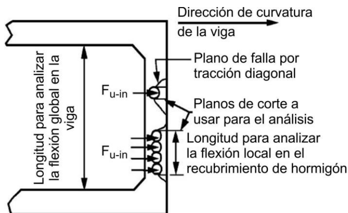
Figura C5.10.4.3.1.1-2 – Solicitaciones en el plano en vigas curvas provocadas por cables curvos en el plano horizontal
