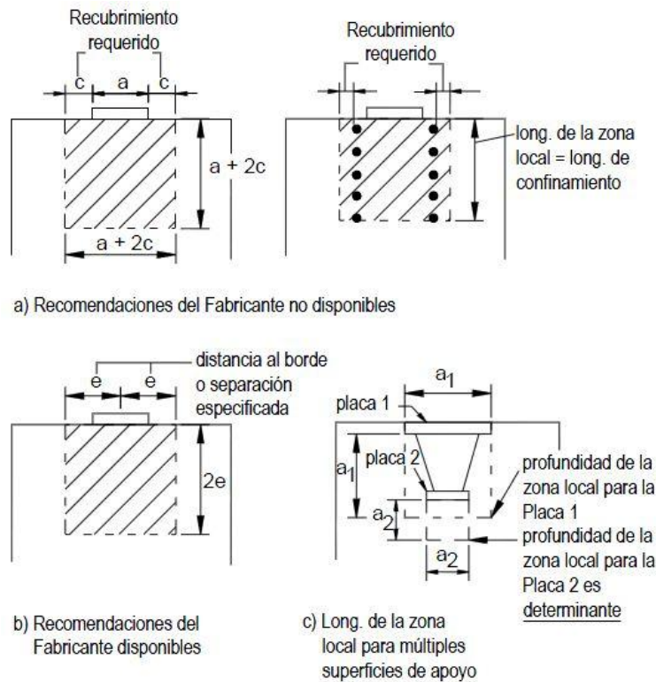
Figura C5.10.9.7.1-1 – Geometría de la zona local
