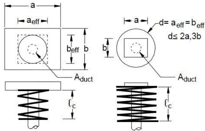
Figura C5.10.9.6.2-3 – Área de apoyo efectiva
