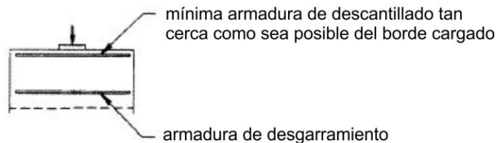
a) Mínima armadura de descantillado
