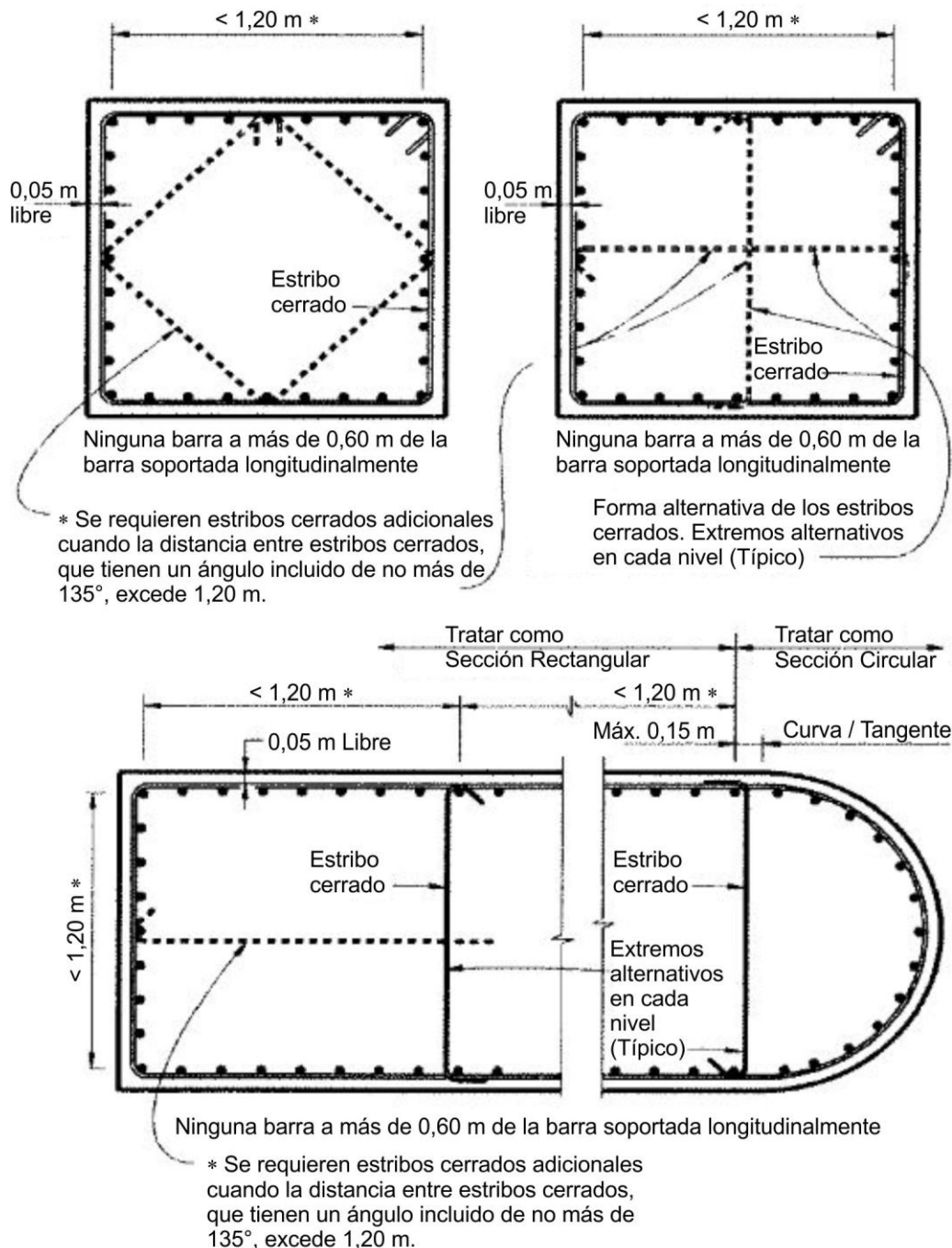
Figura C5.10.6.3-1 – Armado aceptable de los estribos cerrados
