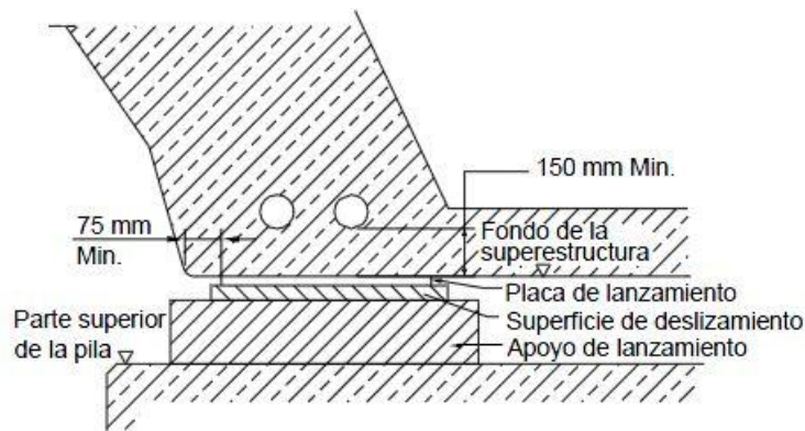
Figura C5.14.2.4.6.3-1 – Ubicación de las placas de lanzamiento
