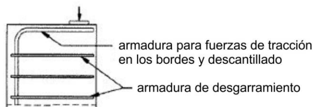
c) Armadura de tracción en los bordes en zonas de anclaje con carga excéntrica
