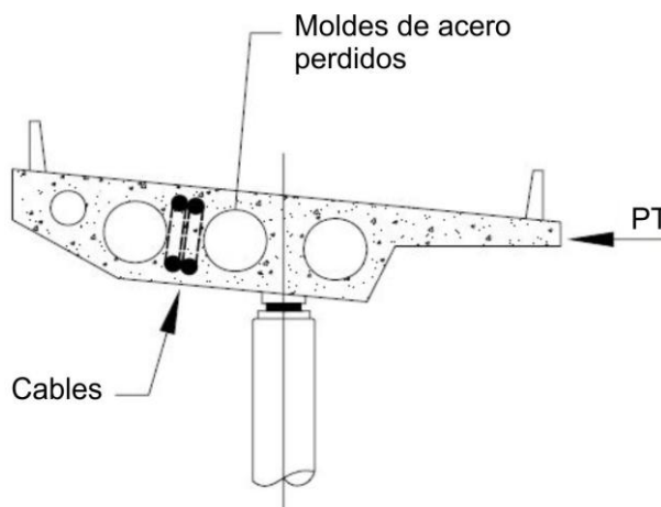
Figura C5.14.4.2.1-1 – Sección transversal de un típico sistema de tablero aligerado
