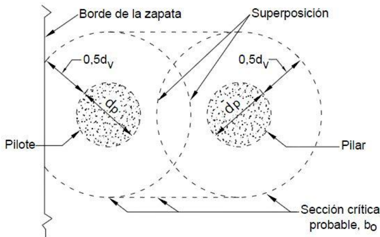
Figura C5.13.3.6.3-1 – Sección crítica modificada para corte con perímetros críticos que se superponen
