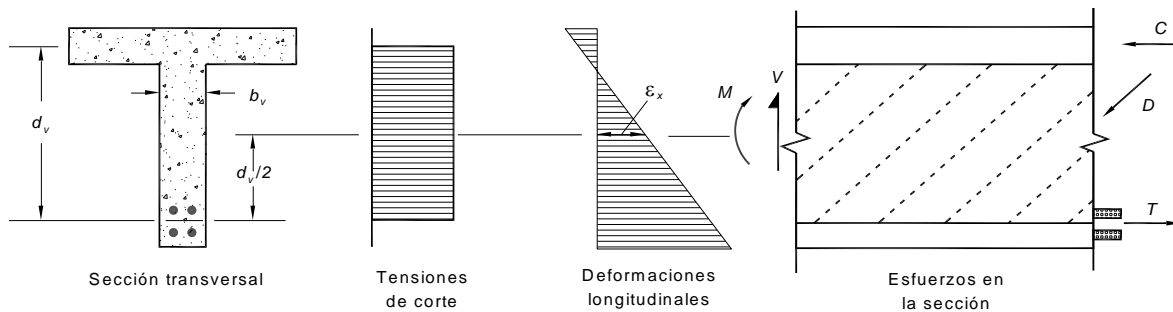
Figura C5.8.3.4.2-2 – Procedimiento más directo para determinar la resistencia al corte de acuerdo con el Artículo 5.8.3.4.2
