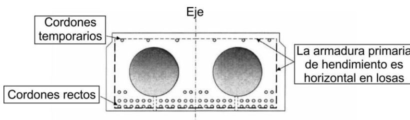
Figura C5.10.10.1-2 – Losa hueca prefabricada
