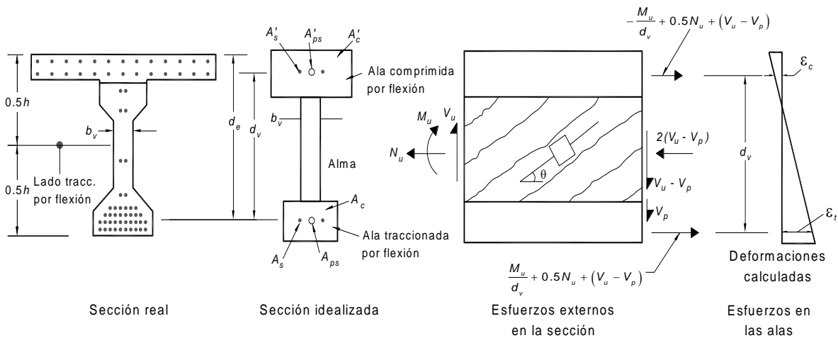
Figura C5.8.3.4.2-3 – Procedimiento de cálculo más preciso para determinar \epsilon_s
