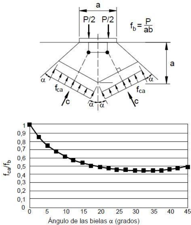
Figura C5.10.9.6.2-1 – Zona local e interfase de las bielas
