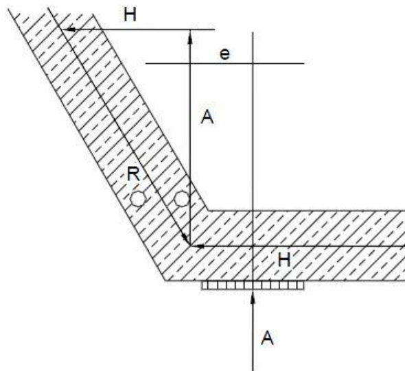
Figura C5.14.2.4.6.3-2 – Reacción excéntrica en las placas de lanzamiento
