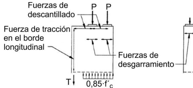
Figura C5.10.9.3.2-3 – Fuerzas de tracción en los bordes
