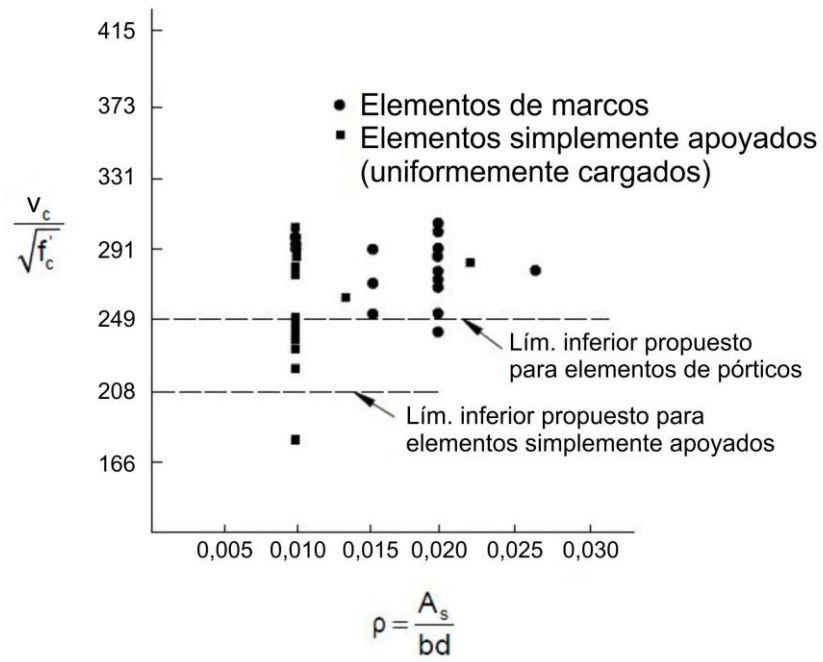
Figura C5.14.5.3-1 – Resultados de ensayos de alcantarillas
