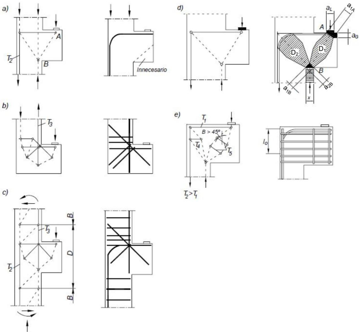
Figura C5.13.2.4.1-1 – Diferentes condiciones de apoyo que conducen a diferentes modelos de bielas y tirantes y diferentes disposiciones de armadura en ménsulas cortas y vigas con resaltos horizontales (Schlaich et al., 1987)
