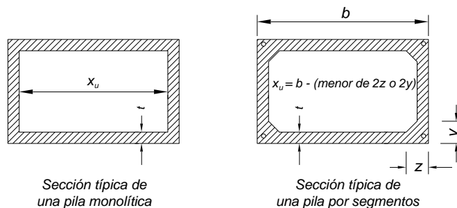
Figura C5.7.4.7.1-1 – Definición de X_u
