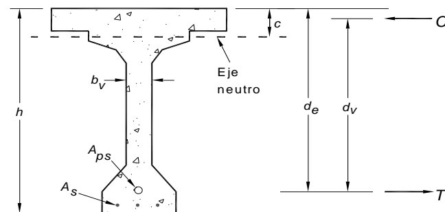
Figura C5.8.2.9-1 – Ilustración de los términos b_v y d_v
