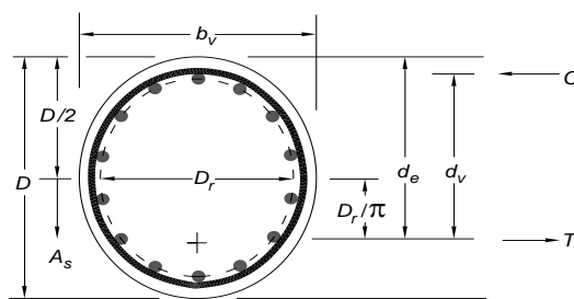
Figura C5.8.2.9-2 – Ilustración de los términos b_v , d_v y d_e para secciones circulares
