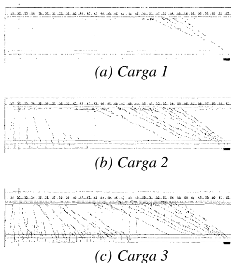
Figura C5.8.3.4.3-1 – Desarrollo de fisuración por corte en una viga bulb-T uniformemente cargada con cargas crecientes; Carga 1 < Carga 2 < Carga 3
