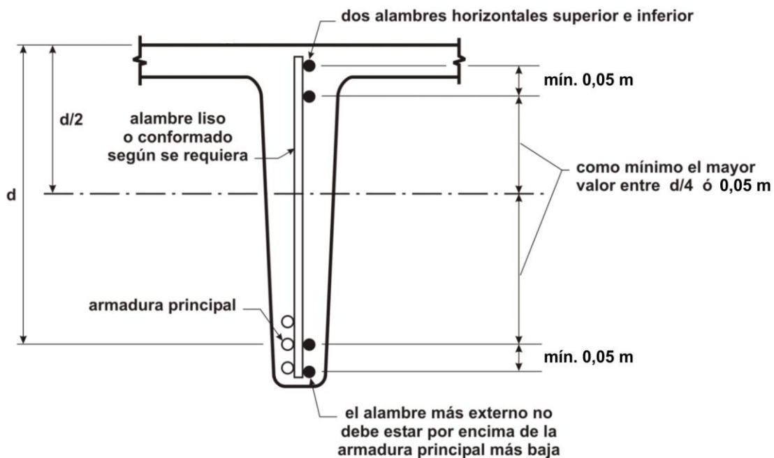
Figura C5.11.2.6.3-1 – Anclaje de la armadura de corte compuesta por un estribo de una rama realizado con malla de acero soldada.
