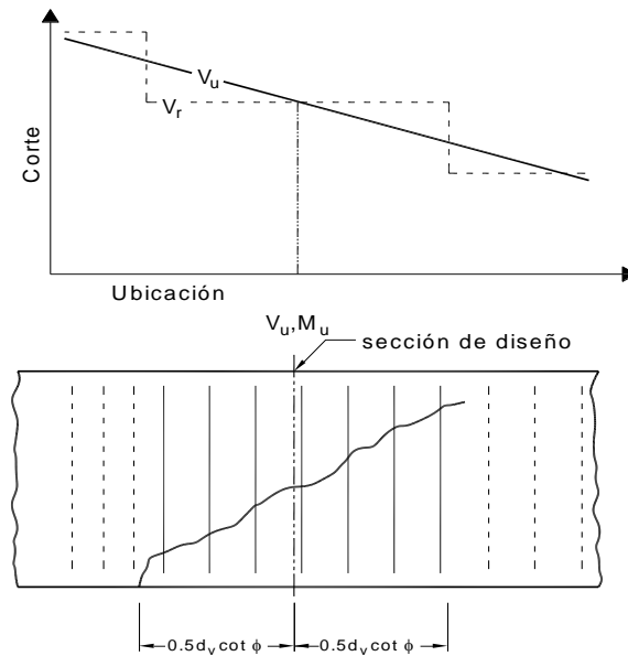
Figura C5.8.3.2-2 – Sección para el diseño simplificado en el caso de cargas aplicadas a la mitad de la profundidad del elemento o por encima de la misma
