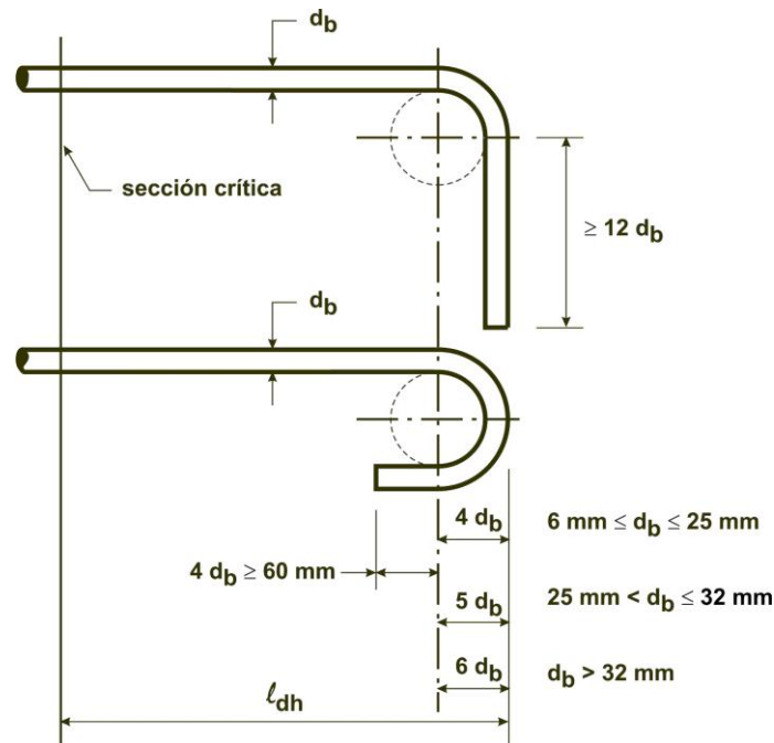
Figura C5.11.2.4-1 – Detalle de los ganchos en las barras y alambres para efectivizar el anclaje de la armadura
