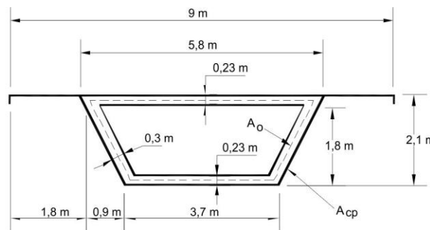
Figure C5.8.2.1-1 – Esquema que muestra los datos usados en el ejemplo de cálculo de A_o incluido a continuación
