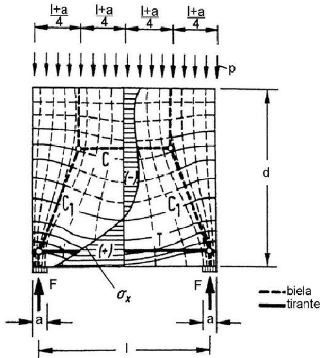
Figura C5.10.9.4.1-1 – Campo de tensiones principales, y superpuesto con el modelo de bielas y tirantes
