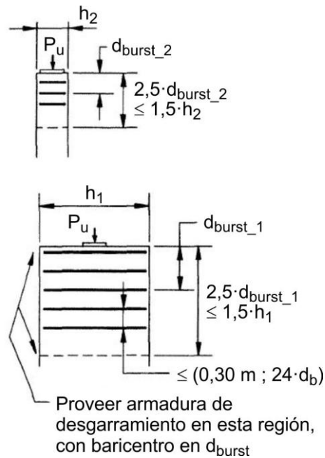
Figura C5.10.9.3.2-1 – Disposición de la armadura de desgarramiento
