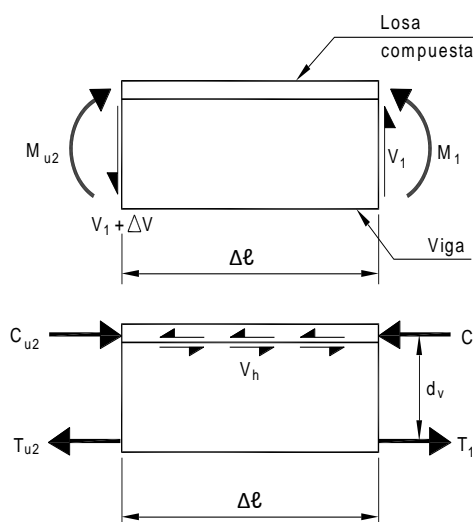
Figura C5.8.4.1-1 – Diagramas de cuerpo libre
