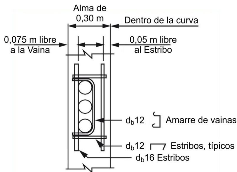
Figura C5.10.4.3.1.2-1 — Detalle de estribo abierto típico y amarre de vainas
