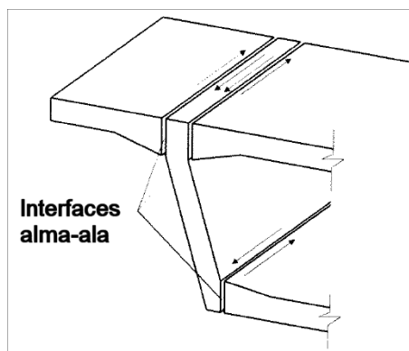
Figura C5.8.4.1-1 – Transferencia de corte longitudinal entre las alas y las almas de los puentes viga tipo cajón
