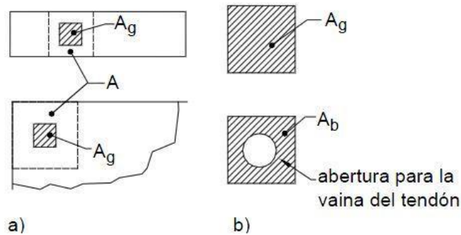
Figura C5.10.9.7.2-1 – Área de la superficie de apoyo de hormigón para la Ecuación 5.10.9.7.2-2
