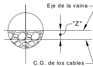
Figura C5.9.1.6-1 – Posición del cable dentro de la vaina
