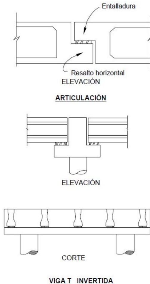
Figura C5.13.2.5.1-1 – Ejemplos de vigas con resaltos horizontales
