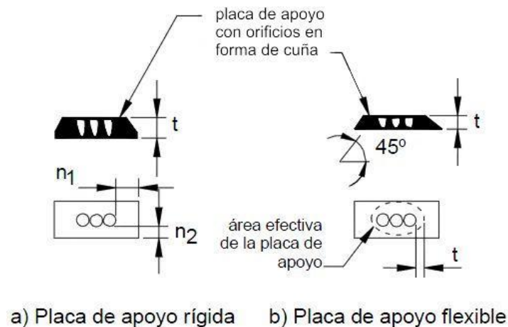
Figura C5.10.9.7.2-3 – Área efectiva de la placa de apoyo para dispositivos de anclaje sin placa de acuñamiento separada
