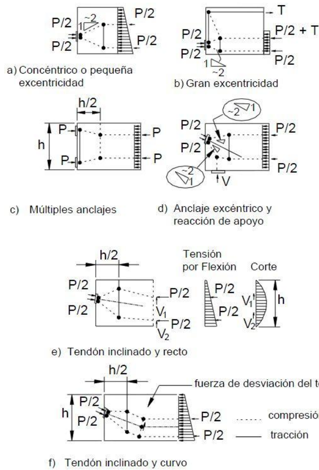
Figura C5.10.9.4.1-2 – Modelos de bielas y tirantes para algunas zonas de anclaje
