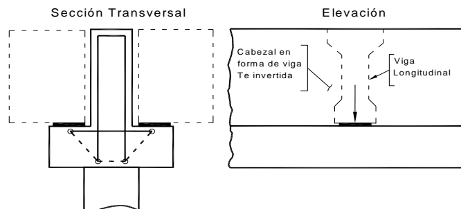
Figura C5.8.3.2-3 – Cabezal consistente en una viga T invertida
