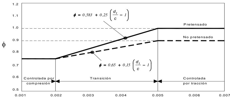
Figura C5.5.4.2.2-1 – Variación de \phi en función de la deformación unitaria neta por tracción \epsilon_t y d/c para armadura f_y = 420 \text{ MPa} y para acero de pretensado
