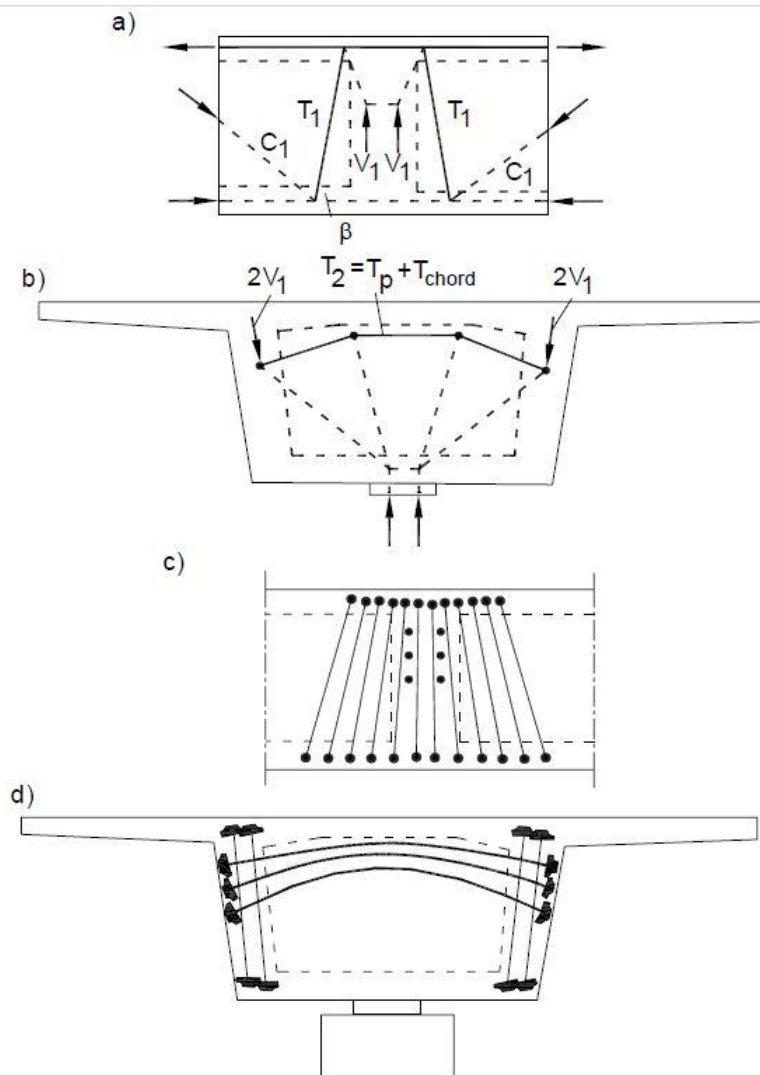
Figura C5.13.2.2-1 – Diafragma de un puente tipo viga cajón: a) Regiones perturbadas y modelo del alma cerca del diafragma; b) Diafragma y modelo; c) y d) Pretensado del alma y del diafragma (Schlaich et al., 1987)
