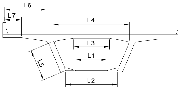
Figura C5.9.4.2.1-1 – Longitudes sugeridas a considerar
