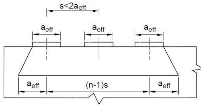
Figura C5.10.9.6.2-2 – Múltiples anclajes poco separados
