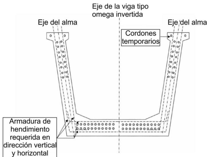
Figura C5.10.10.1-1 – Viga tipo omega invertida prefabricada
