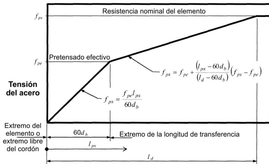
Figura C5.11.4.2-1 – Relación teórica entre la tensión del acero y la distancia desde el extremo libre del cordón.
