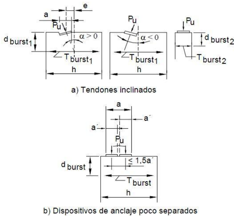
Figura C5.10.9.6.3-1 – Simbología utilizada en las Ecuaciones 5.10.9.6.3-1 y 5.10.9.6.3-2
