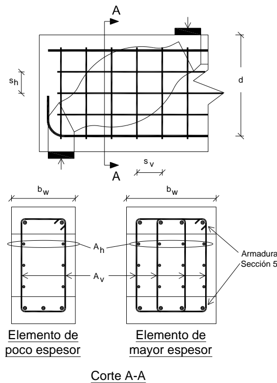
Figura C5.6.3.6-1 – Distribución de la armadura para limitar la fisuración en una biela comprimida
