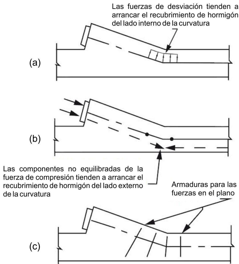
Figura C5.10.4.3.1.1-1 – Fuerzas en el plano en un taco para anclaje
