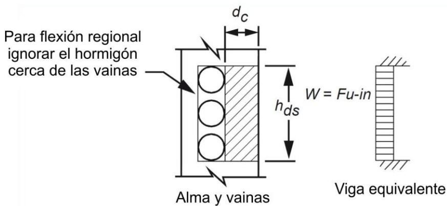
Figura C5.10.4.3.1.3-1 — Recubrimiento de hormigón de una viga hipotética sin armar
